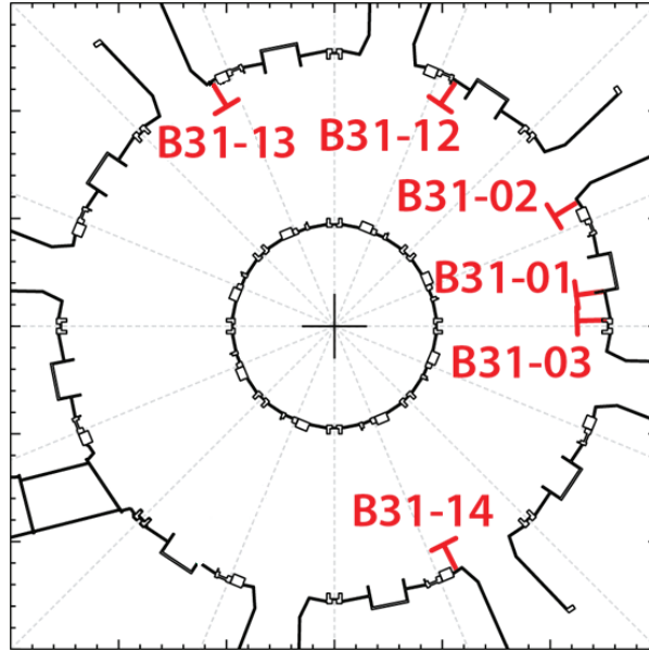
1.3. ábra. Az ASDEX Upgrade tokamak középsőjében elhelyezett mágneses szondák pozícióját szemléltető sematikus ábra felülnézetben.
