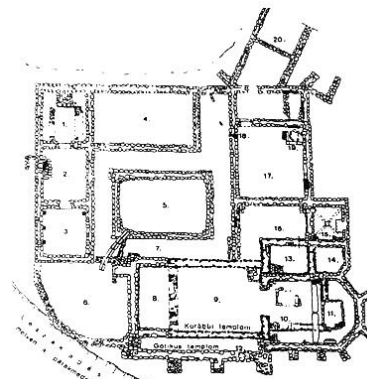
33. A felnémeti kolostor alaprajza 29
