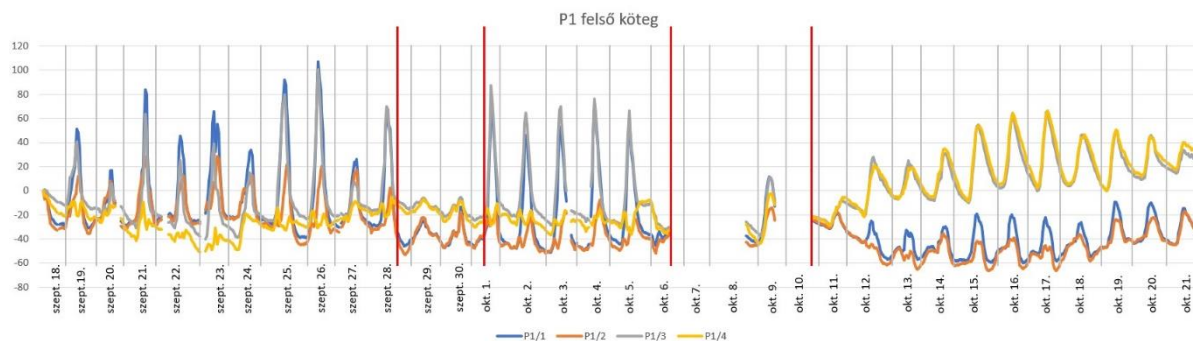
6.7. ábra: P1 felső köteg mérési eredményei (ősz).
