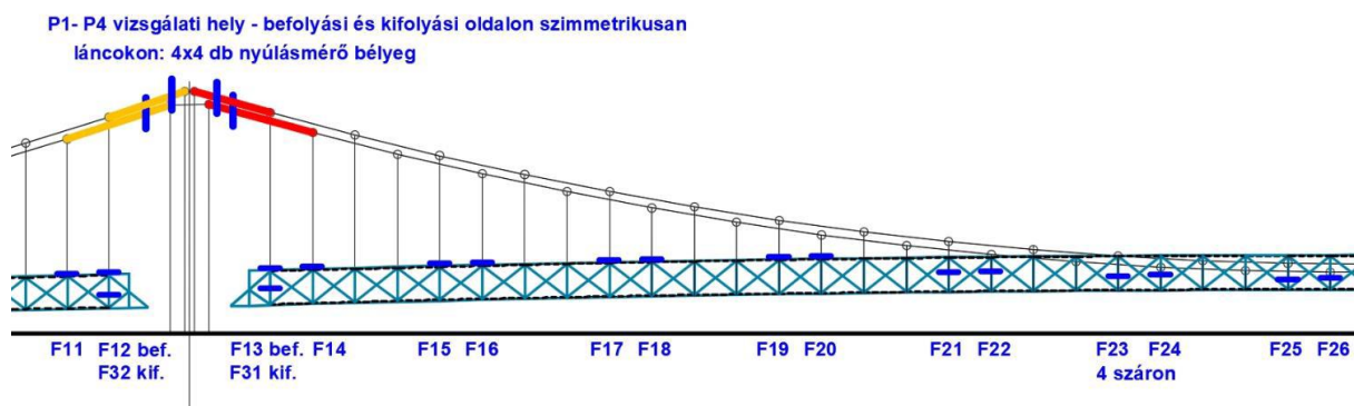
5.2. ábra: Nyúlásmérési helyek globális helyzete II.
