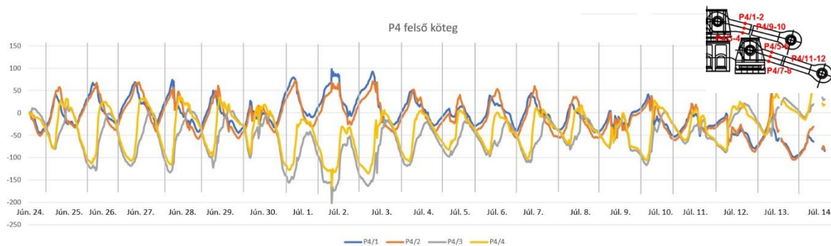
6.30. ábra: P4 felső köteg mérési eredménye (nyár).
