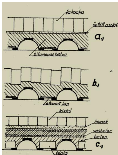
3.12. ábra: A fakockaburkolat romlása [5].
