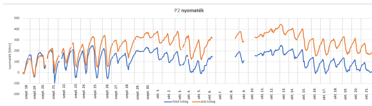
6.18. ábra: P2 mérőhelyen kialakult nyomaték.
