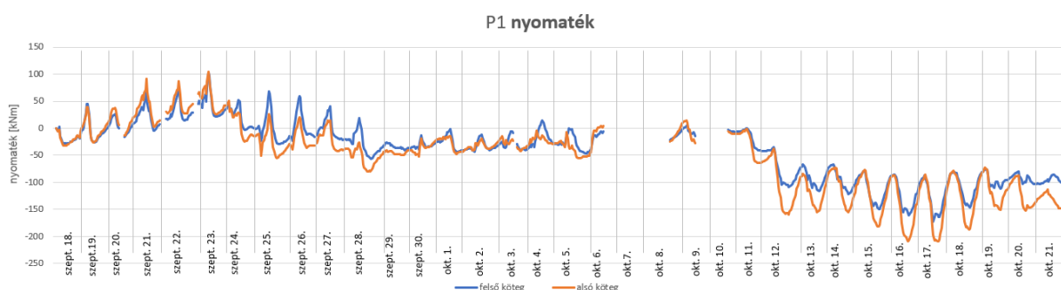
6.9. ábra: P1 mérőhelyen kialakult nyomaték.
