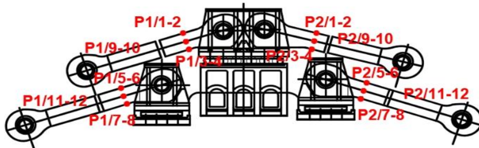
5.11. ábra: Nyúlásmérő bélyegek elhelyezkedése a P1 és P2 mérőhelyeken.
