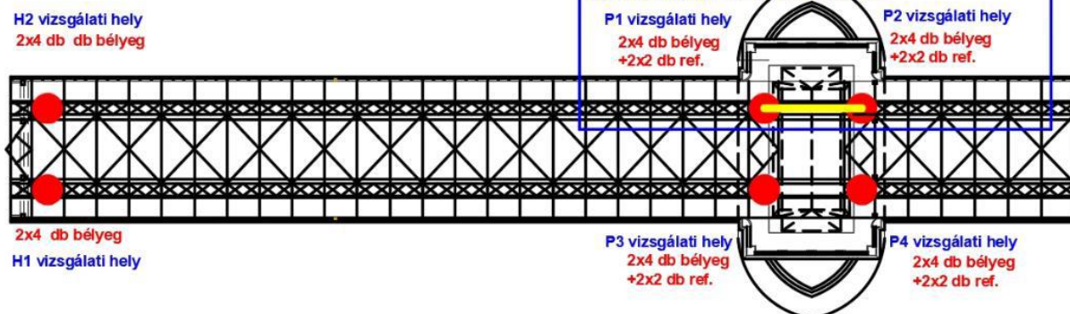
5.4. ábra: Nyúlásmérési helyek globális helyzete IV.
