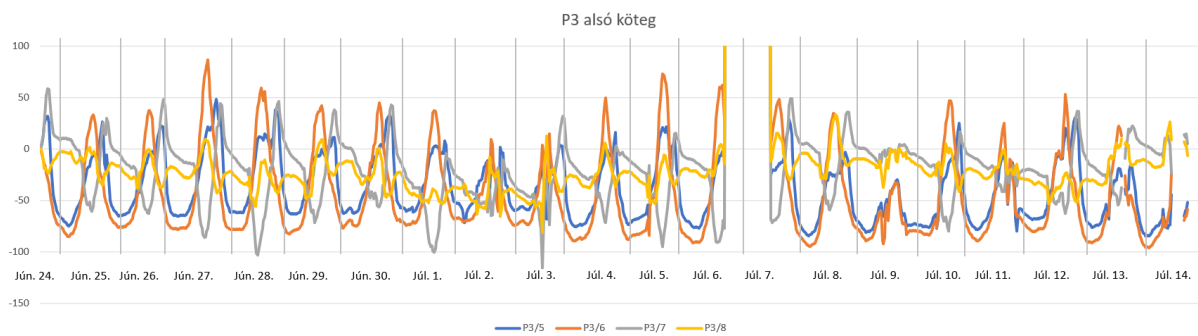
6.23. ábra: P3 alsó köteg mérési eredménye (nyár) – korrigált.
