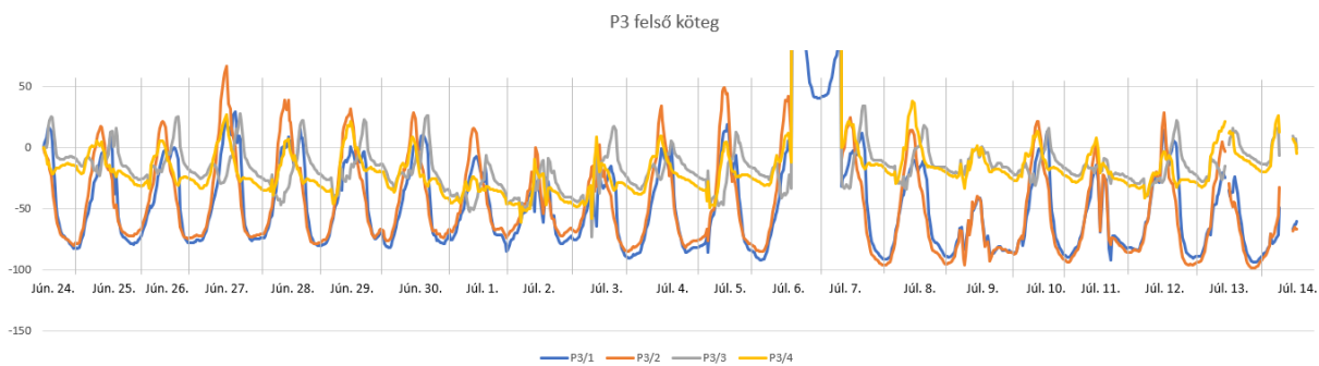
6.22. ábra: P3 felső köteg mérési eredménye (nyár) – korrigált.
