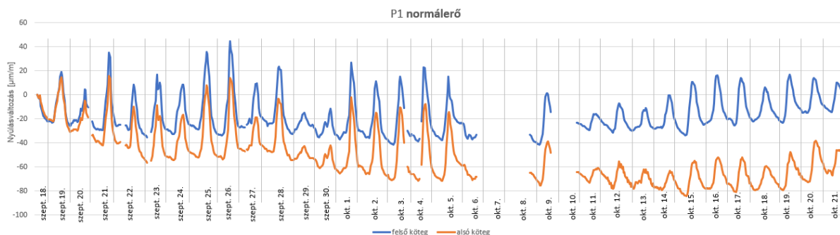
6.10. ábra: Normál feszültség bemutatása a szélső szálak átlagából.
