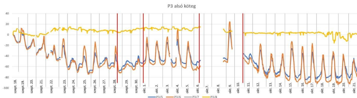
6.26. ábra: P3 alsó köteg mérési eredménye (ősz).
