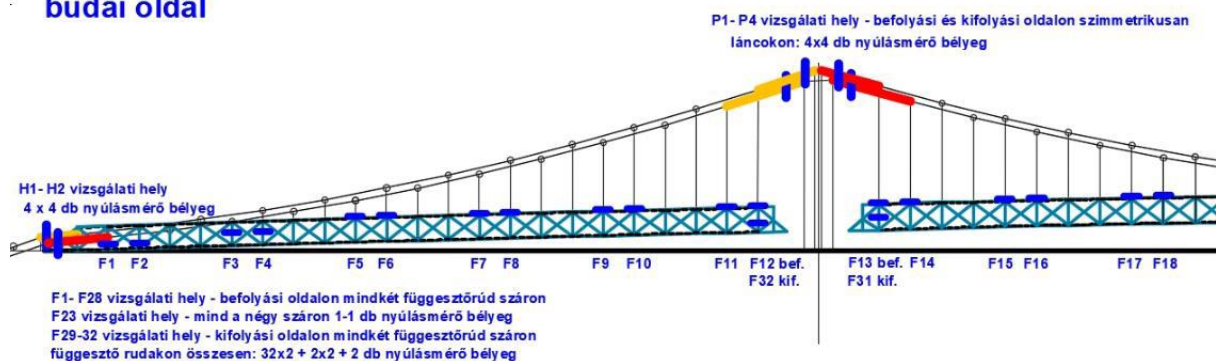
5.1. ábra: Nyúlásmérési helyek globális helyzete I.
