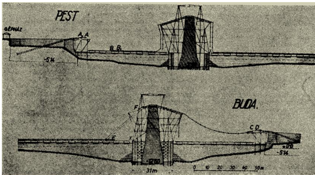
3.4. ábra: Láncok szerelése [5].
