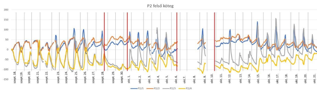
6.16. ábra: P2 felső köteg mérési eredménye (ősz).
