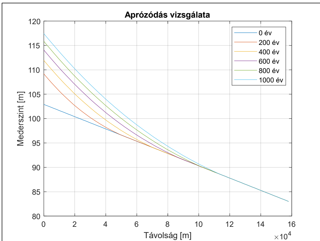
29. ábra: Mederszintek változása 1000 év alatt egyenletes vízmozgás esetén az aprózódást is figyelembe véve
