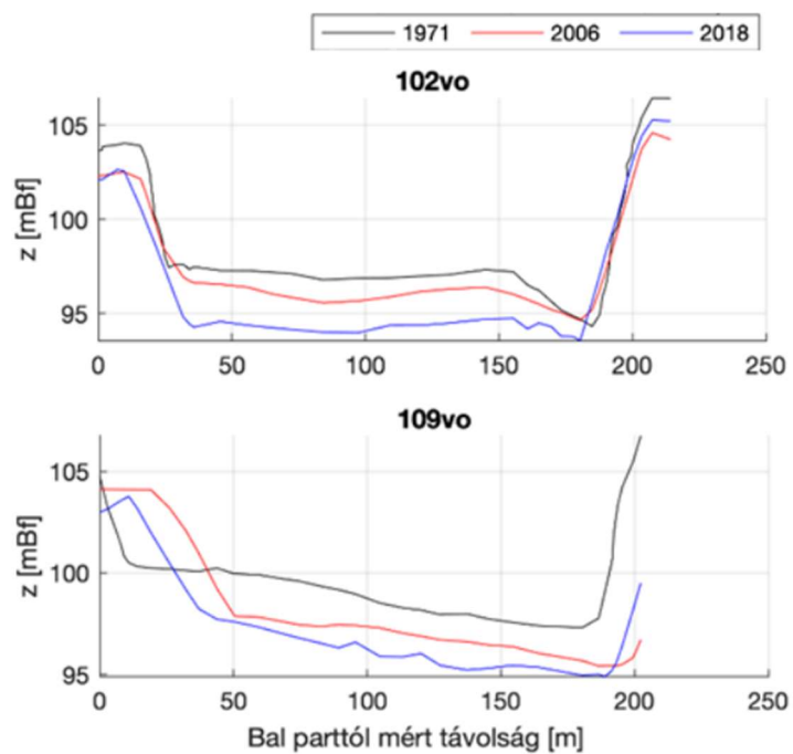
8. ábra: Jellemző keresztmetszvények Barcs környezetében 3 különböző időszakból (Forrás: BME VVT, 2020)
