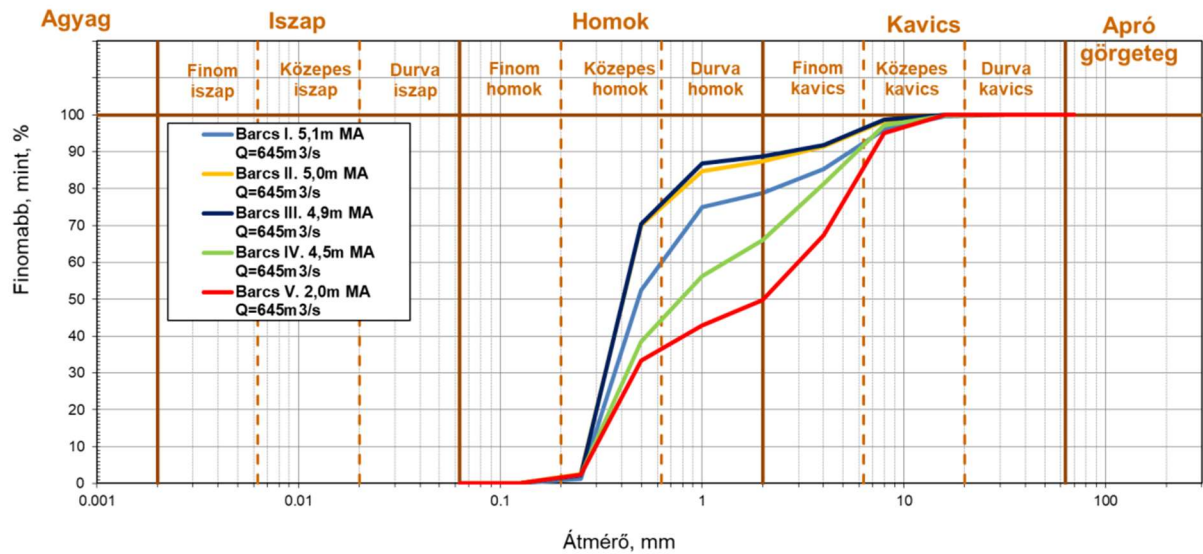
14. ábra: Barcs mederanyag szemösszetételi görbe (Forrás: BME VVT, 2019)
