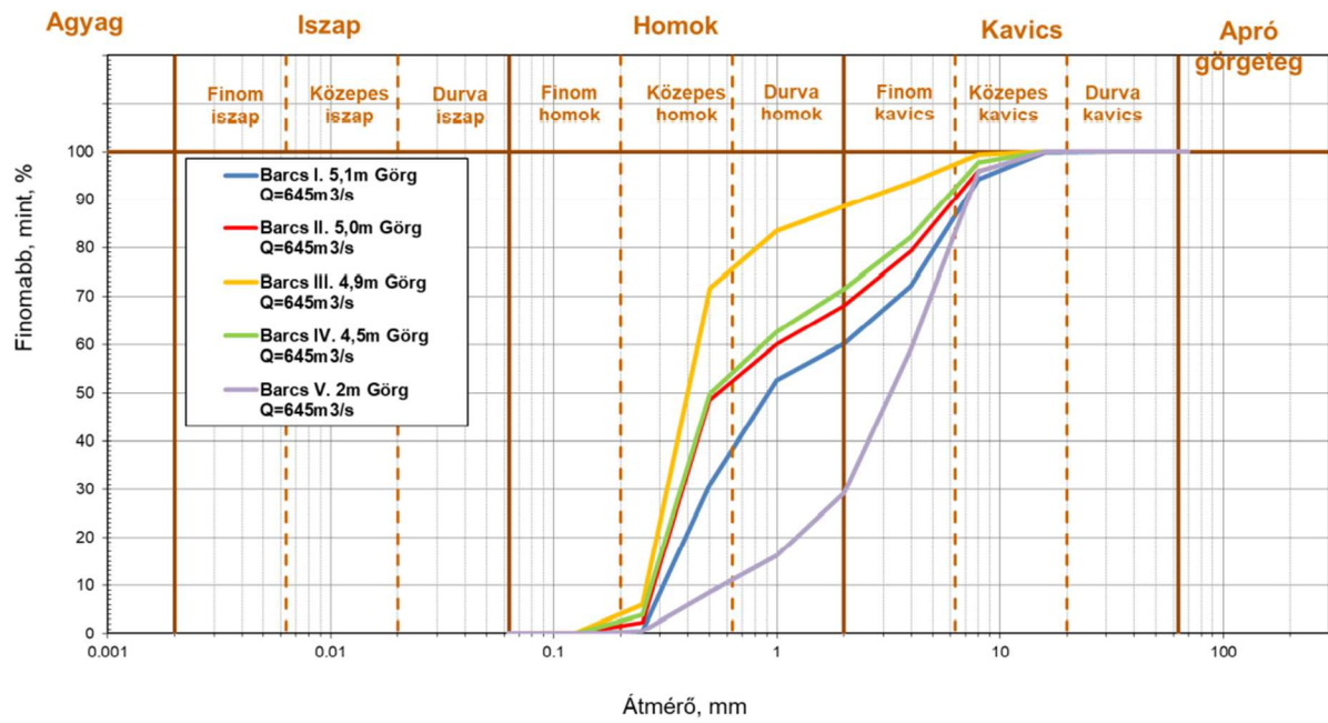
13. ábra: Barcs gőrgetett hordalék szemeloszlási görbe (Forrás: BME VVT, 2019)
