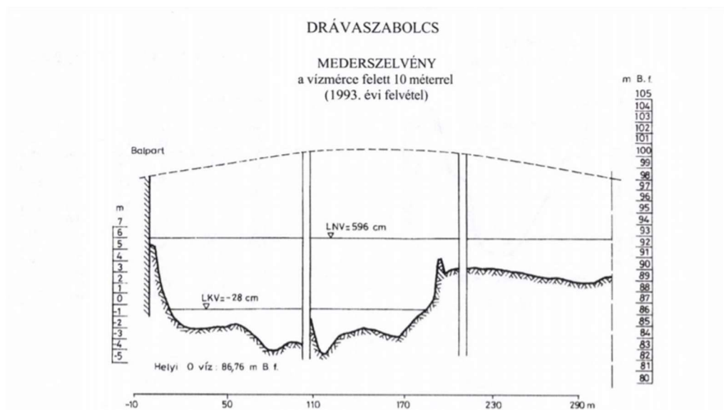
6. ábra: Drávaszabolcs 1993-es mederfelvételi ábrája (Forrás: 1994. évi Vízirajzi Évkönyv)
