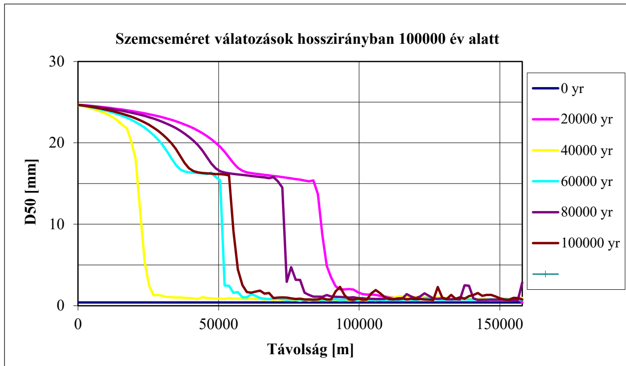
39. ábra: Wilcock és Crowe modell 100000 éves átlagos szemátmérő eredményei az Őrtilos-Drávaszabolcs szakaszán
