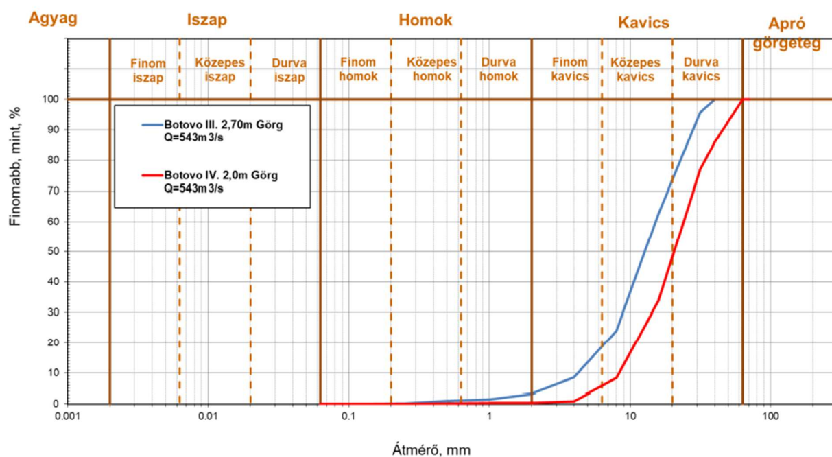
11. ábra: Örtilos gőrgőteg hordalék szemeloszlási görbe (Forrás: BME VVT, 2019)
