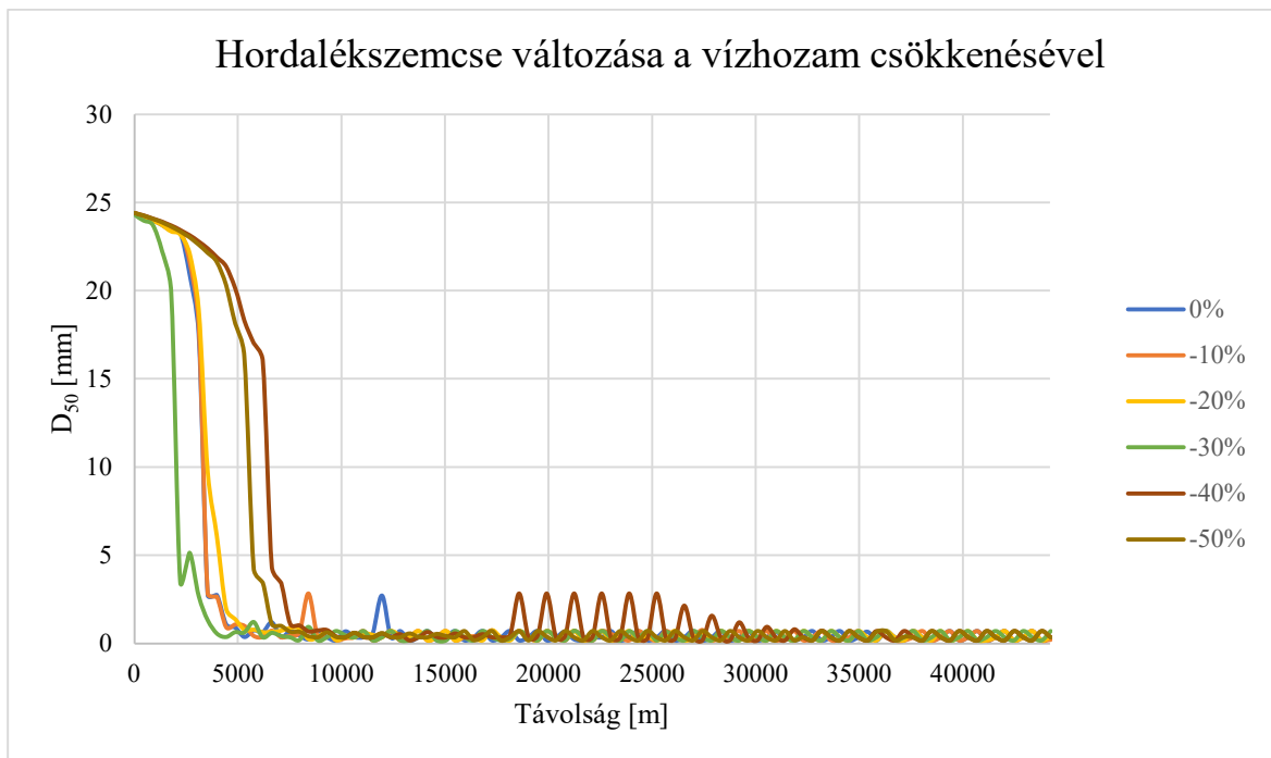
41. ábra: Hordalék-szemcseméret változások a vízhozam csökkenésének függvényében
