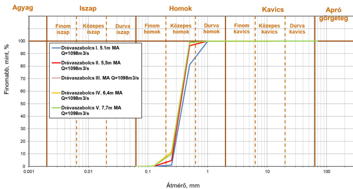
16. ábra: Drávaszabolcs mederanyag szemeloszlási görbe (Forrás: BME VVT, 2019)
