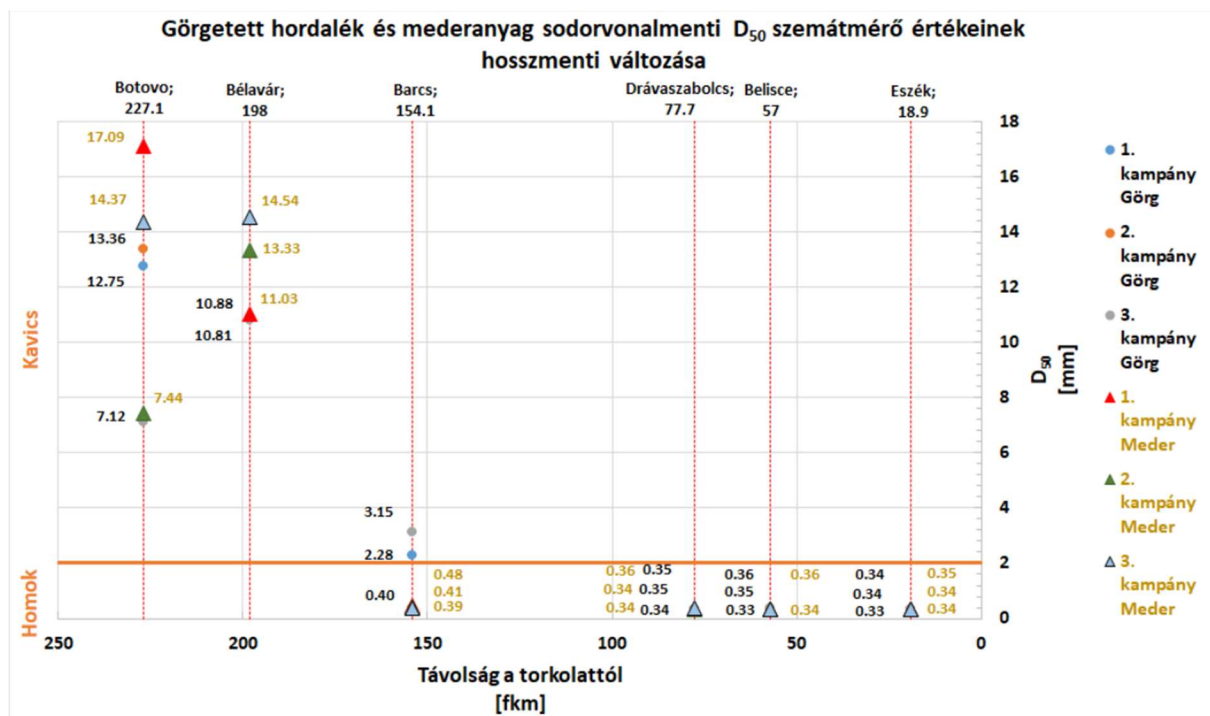
36. ábra: Görgetett hordalék és mederanyag hosszmenti változása (Forrás: BME VVT, 2019)
