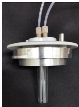
25. ábra: Folyamatos áramlási cella
