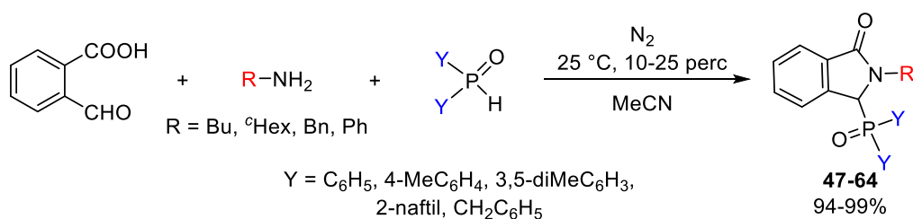
26. ábra: Izoindolinon-foszfin-oxidok előállítása Kabachnik–Fields-reakciót követő gyűrűzárással
