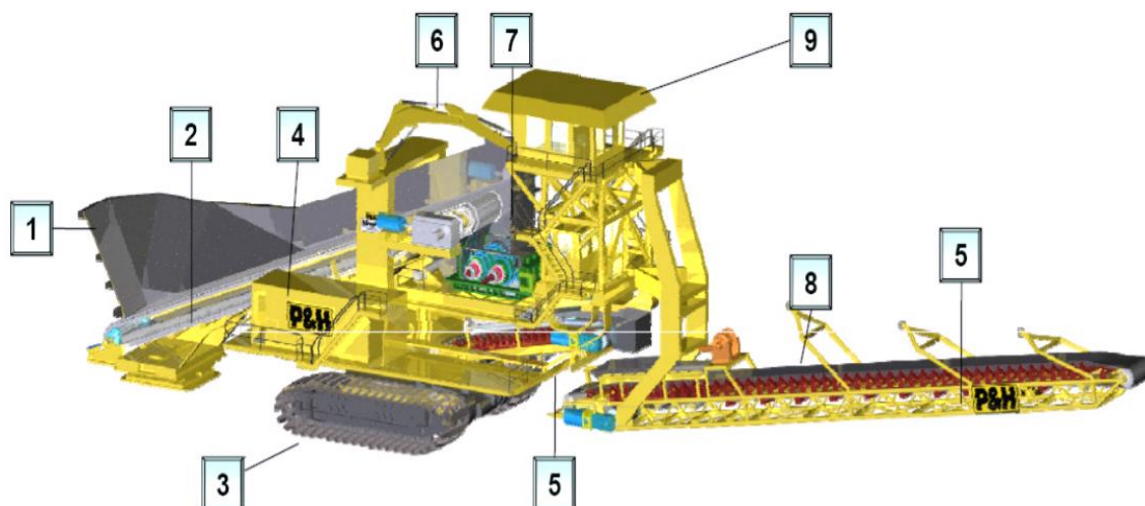
2. ábra: Egy FMIPCC törő felépítése. Az eszközökben többféle törőgép is lehet, nemcsak hengertörő.
