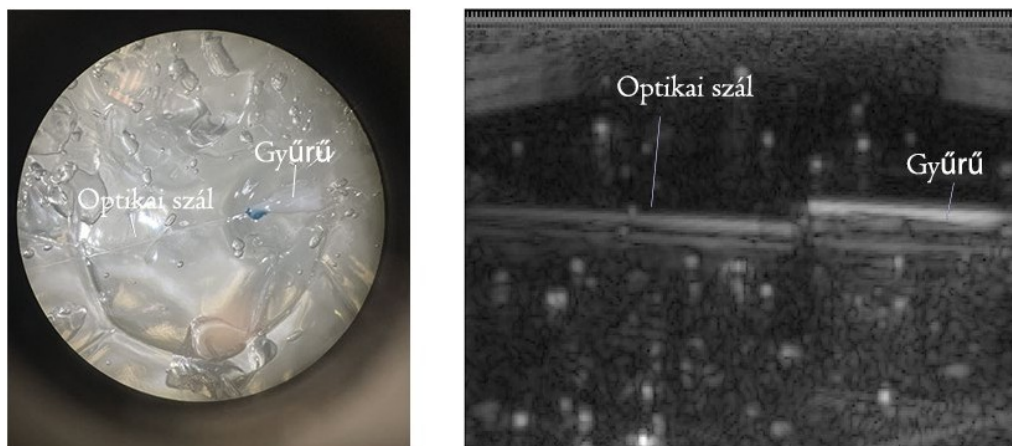
16. ábra - Ultrahang zselébe mártott 50 \mu\text{m} -es optikai szál képe fénymikroszkóp alatt (bal oldali kép), valamint ultrahang képalkotással vizsgálva (jobb oldali kép).
