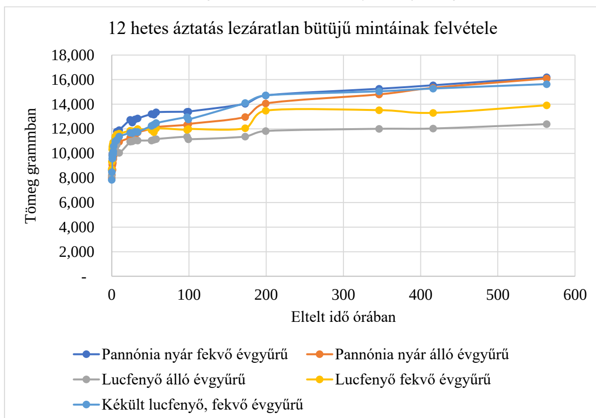
6/2. diagram 12 hetes áztatás lezáratlan bütűjű minták felvételi görbéi
