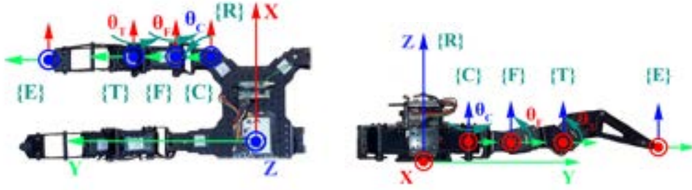
2.3. ábra. Egy tetszőleges láb esetén a robothoz, a csuklókhöz és az effektorhoz rögzített koordináta rendszerek ( \{R\}, \{C\}, \{F\}, \{T\}, \{E\} ) és azok elforgatási szögei ( \theta_{C,F,T} ), ezek színei megegyeznek a tengely színével, mely körül történik az elforgatás. Bal: Felülnézet, a coxa csuklók elfordulása mindig az xOy síkban történik, Oz tengely körül. Jobb: Az x tengely irányából nézve a femur csuklók elfordulása mindig az előzőleg meghatározott koordinátarendszerek yOz síkjaiban történik, Ox tengely körül.
