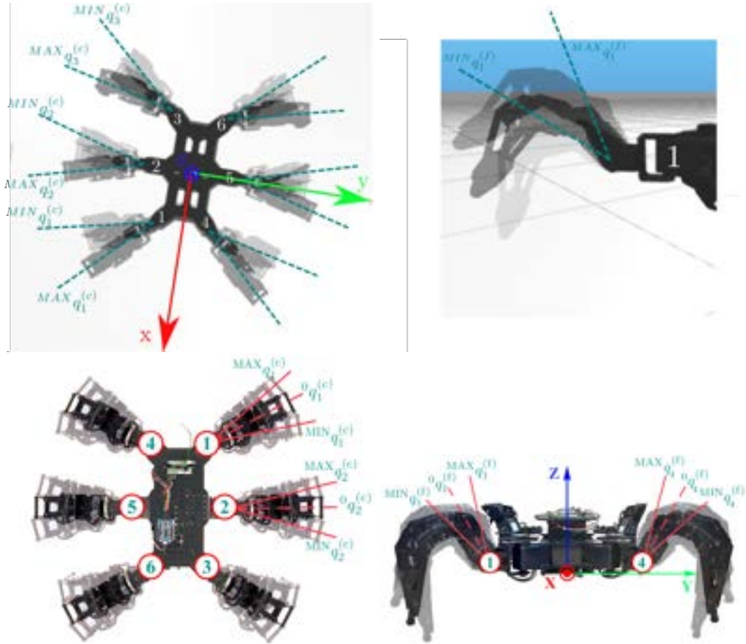
2.2. ábra. A robot coxa- és femurszögeinek határai a szimulációs környezetben ( felső sor ) valamint a valódi robot ( alsó sor ) esetében: a [\text{MIN}_{q_i}^{(c)}, \text{MAX}_{q_i}^{(c)}] és [\text{MIN}_{q_i}^{(f)}, \text{MAX}_{q_i}^{(f)}] intervallumok a hatlábú roboton bejelölve. Az i a robot lábait számláló index. A robothoz csatolt koordinátarendszer jobbsodrású. Bal: A robot lábainak számozása és a coxa csuklók elfordulási intervallumai \text{MAX}_{q_i}^{(c)} - \text{MIN}_{q_i}^{(c)} = \pi/6 . Jobb: \text{MAX}_{q_i}^{(f)} - \text{MIN}_{q_i}^{(f)} = \pi/5 .
