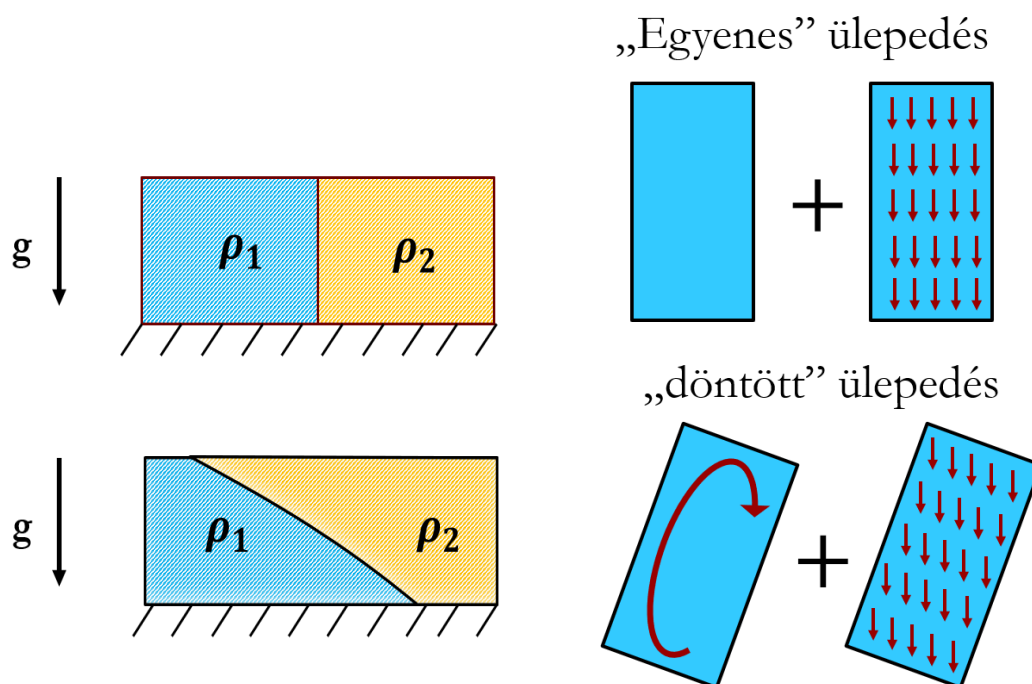
(a) Örvénylés kialakulása két különböző sűrűségű folyadék határán. (b) Az örvénylés hajtóereje a zárt ülepitőben.
