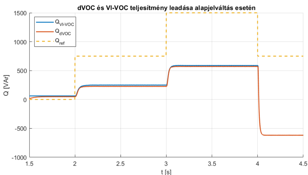
18. ábra: Inverteres egység meddőteljesítmény betáplálása alapjelváltozás és szigetüzembe kerülés hatására
