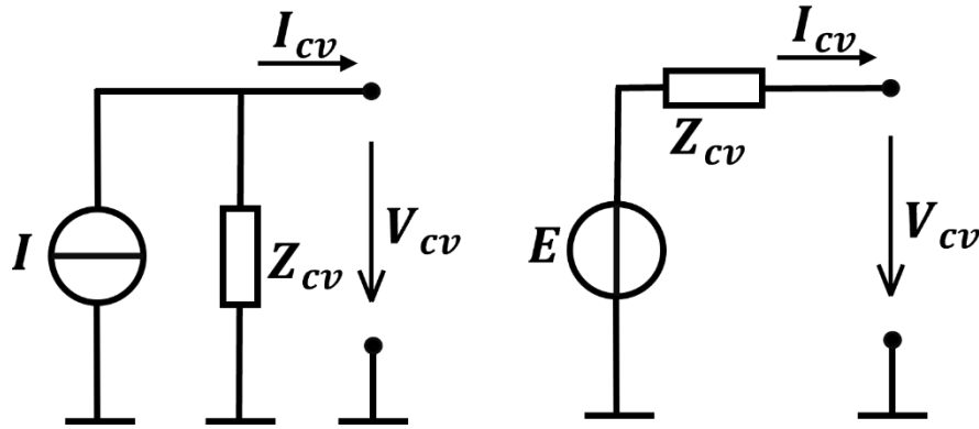
1. ábra: GFL (bal) és GFM (jobb) inverterek egyszerű helyettesítőképei
