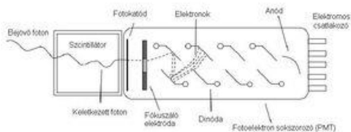
2. ábra Szcintillációs detektor felépítése, forrás: [26]
