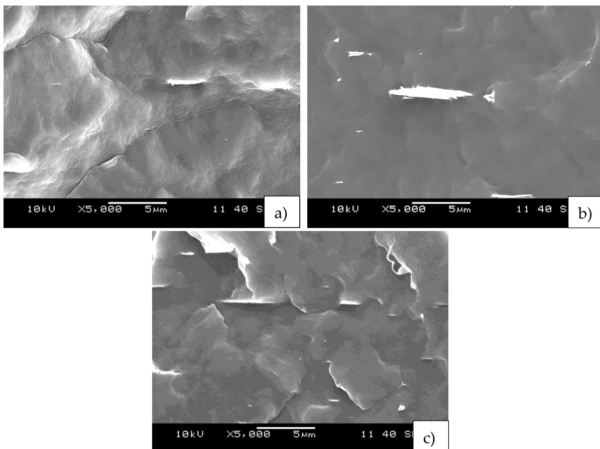
16. ábra: SEM-felvételek a különböző koncentrációban talkumot tartalmazó fóliákról (a: 0,5 m%, b: 1,0 m%, c: 1,5 m%)
