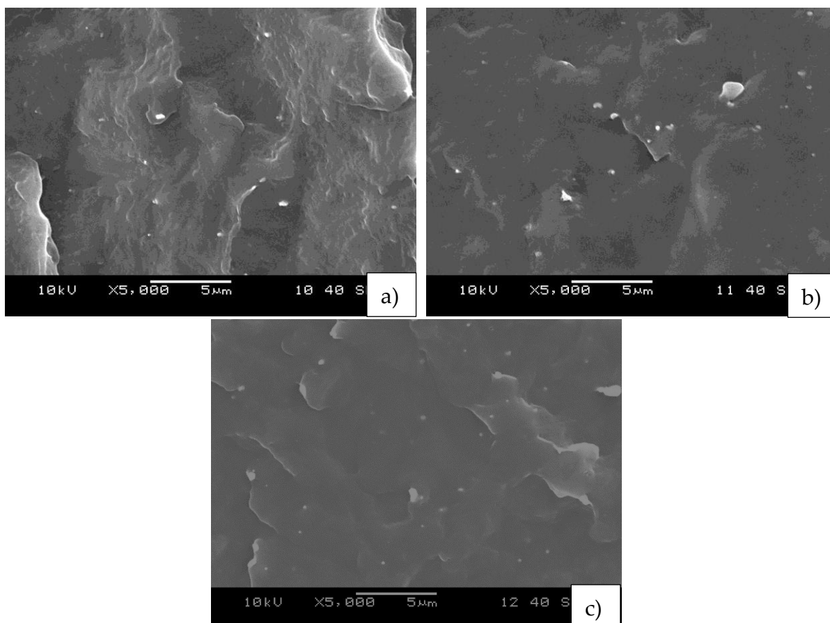
18. ábra: SEM-felvételek a különböző koncentrációban \text{TiO}_2 -t tartalmazó fóliákról (a: 0,5 m%, b: 1,0 m%, c: 1,5 m%)
