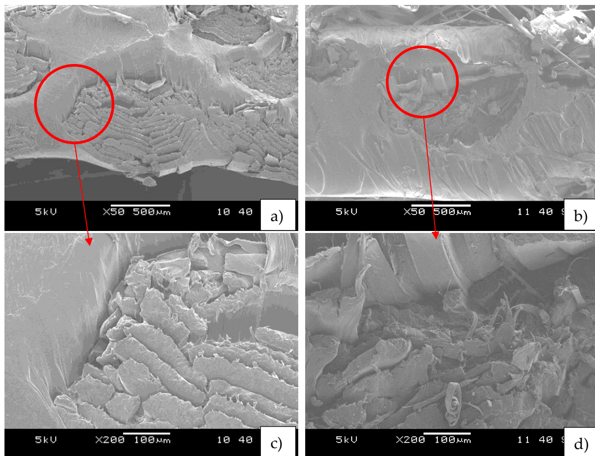
25. ábra: A kompozitokról készült SEM-felvételek (a és c: vágási felület, b és d: töretfelület)
