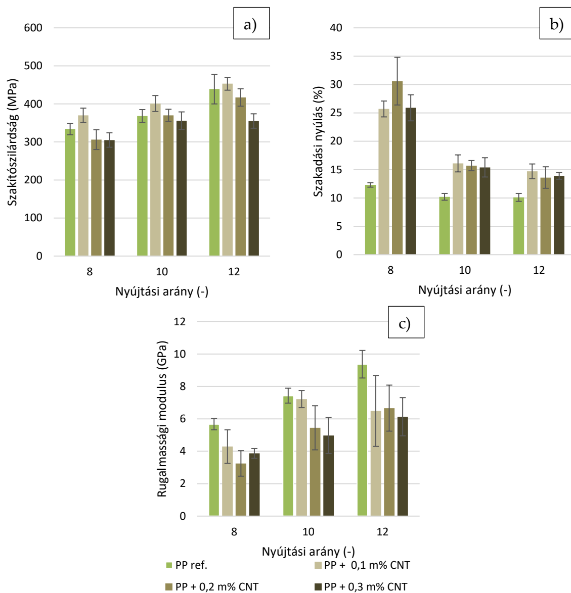
21. ábra: A CNT-vel adalékolt PP fóliák szilárdsági tulajdonságai a CNT mennyisége és a nyújtási arány függvényében (a: szakítószilárdság, b: szakadási nyúlás, c: rugalmassági modulus)
