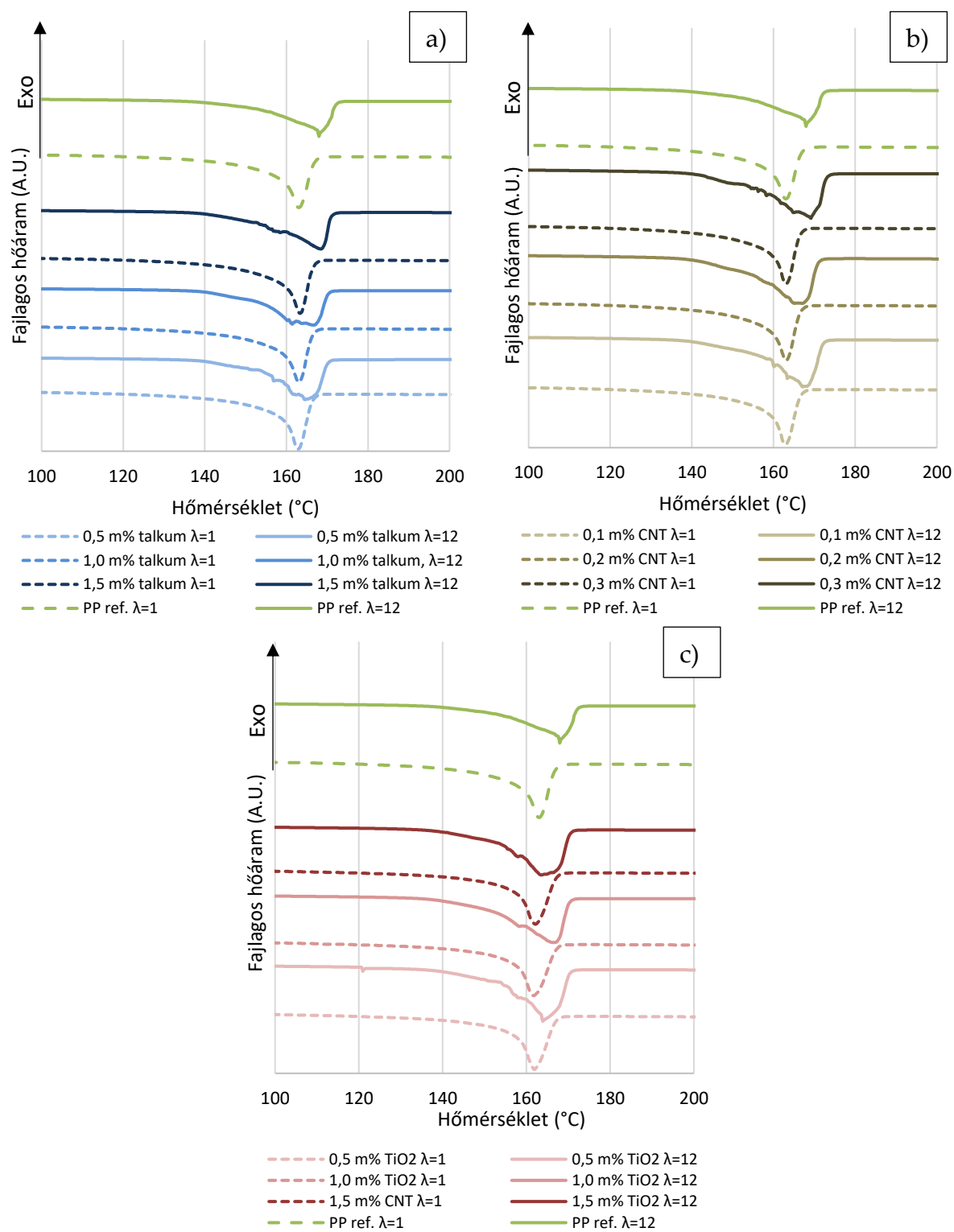
19. ábra: Az egyes kompaundokhoz és a vizsgált nyújtási arányokhoz tartozó DSC-görbék (a: talkum, b: CNT, c: TiO 2 )
