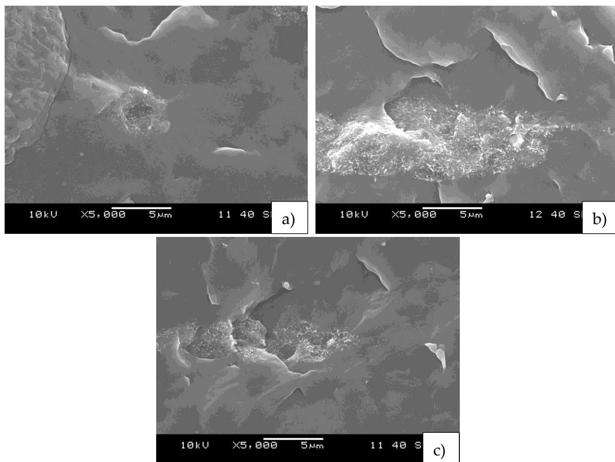
17. ábra: SEM-felvételek a különböző koncentrációban CNT-t tartalmazó fóliákról (a: 0,1 m%, b: 0,2 m%, c: 0,3 m%)
