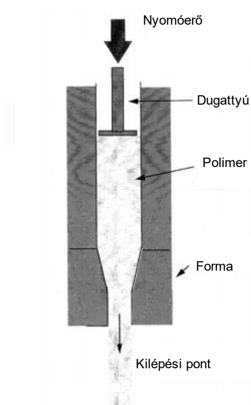
5. ábra: A szilárd állapotú extrúzió [3]
