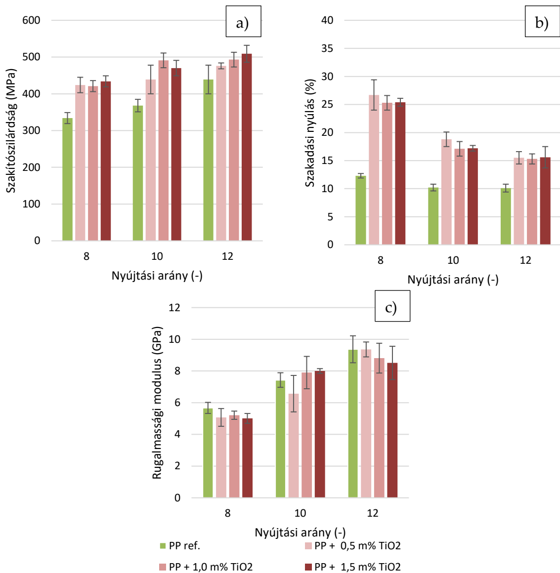
22. ábra: A TiO 2 -vel adalékolt PP fóliák szilárdsági tulajdonságai a TiO 2 mennyisége és a nyújtási arány függvényében (a: szakítószilárdság, b: szakadási nyúlás, c: rugalmassági modulus)
