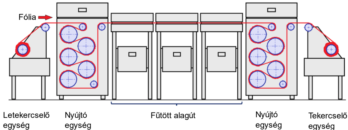
9. ábra: A fólianyújtósor felépítése
