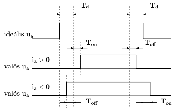
(b) Az a fázis feszültsége ideális és holtidős esetben, figyelembe véve a tranzisztorok be- és kikapcsolási idejét
