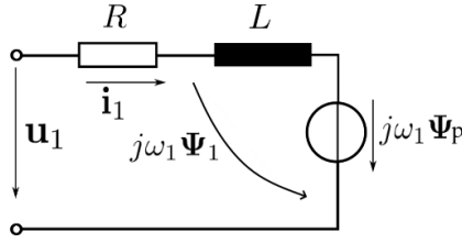
2. ábra. PMSM motor helyettesítő áramköri képe [13]
