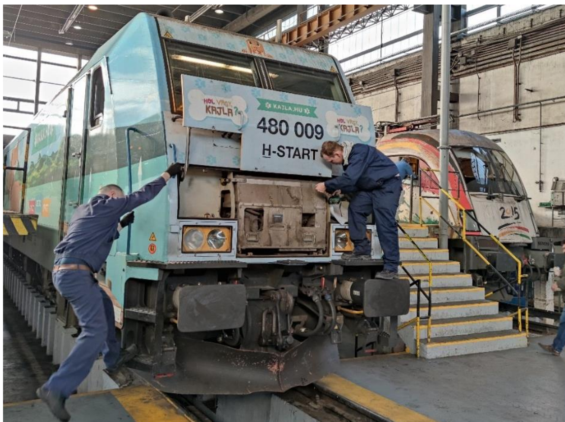
3. melléklet 2. ábra: TRAXX mozdony kinyitott orrburkolattal
