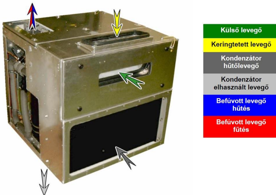
3. melléklet 16. ábra: A klímaegység levegőelosztása (forrás: FLIRT felhasználói kézikönyv)
