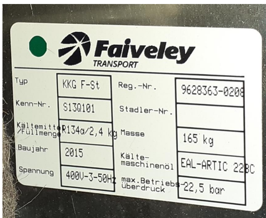
3. melléklet 17. ábra: FLIRT motorvonat klímaberendezés adattáblája
