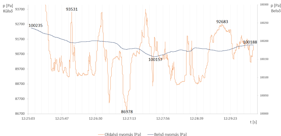
26. ábra: Vectron mozdony mérési adatainak egy másik részlete {2. melléklet 2. ábra}
