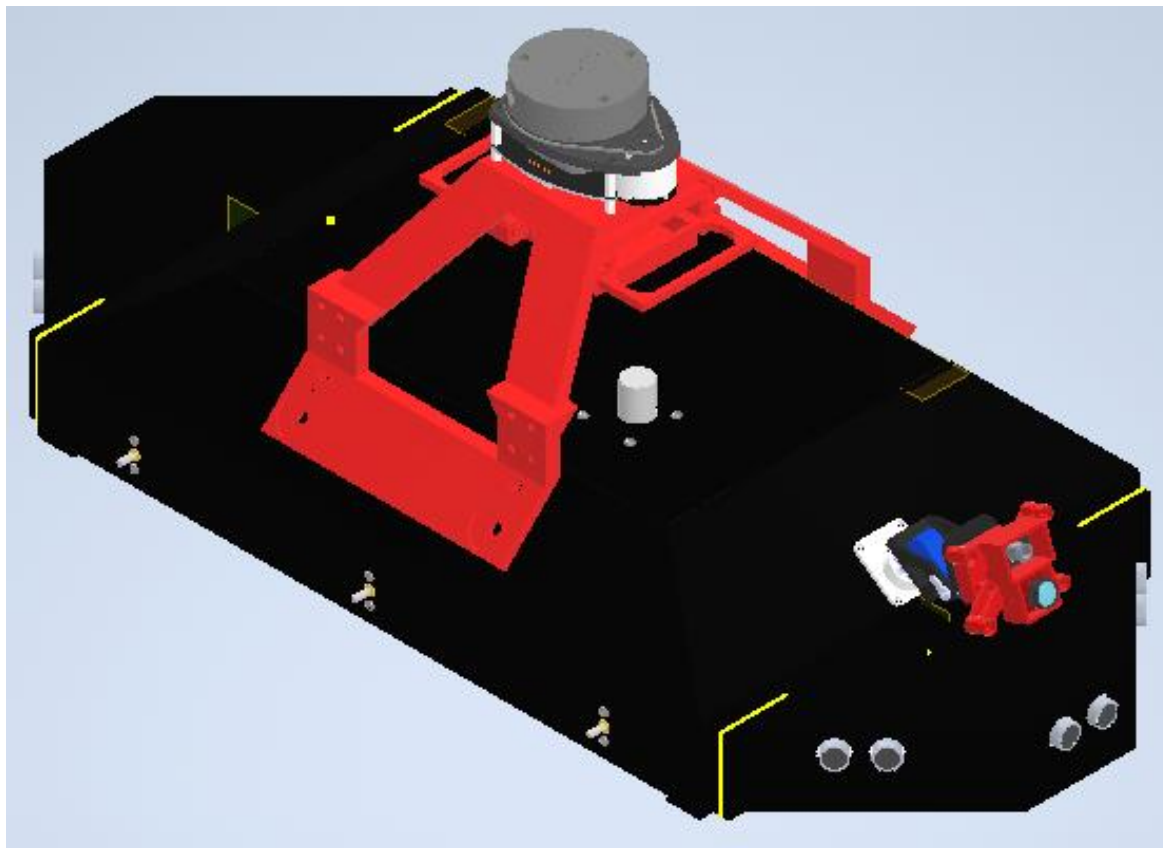
HEAT SPOTTER ház, a főbb külső műanyag elemekkel 11
