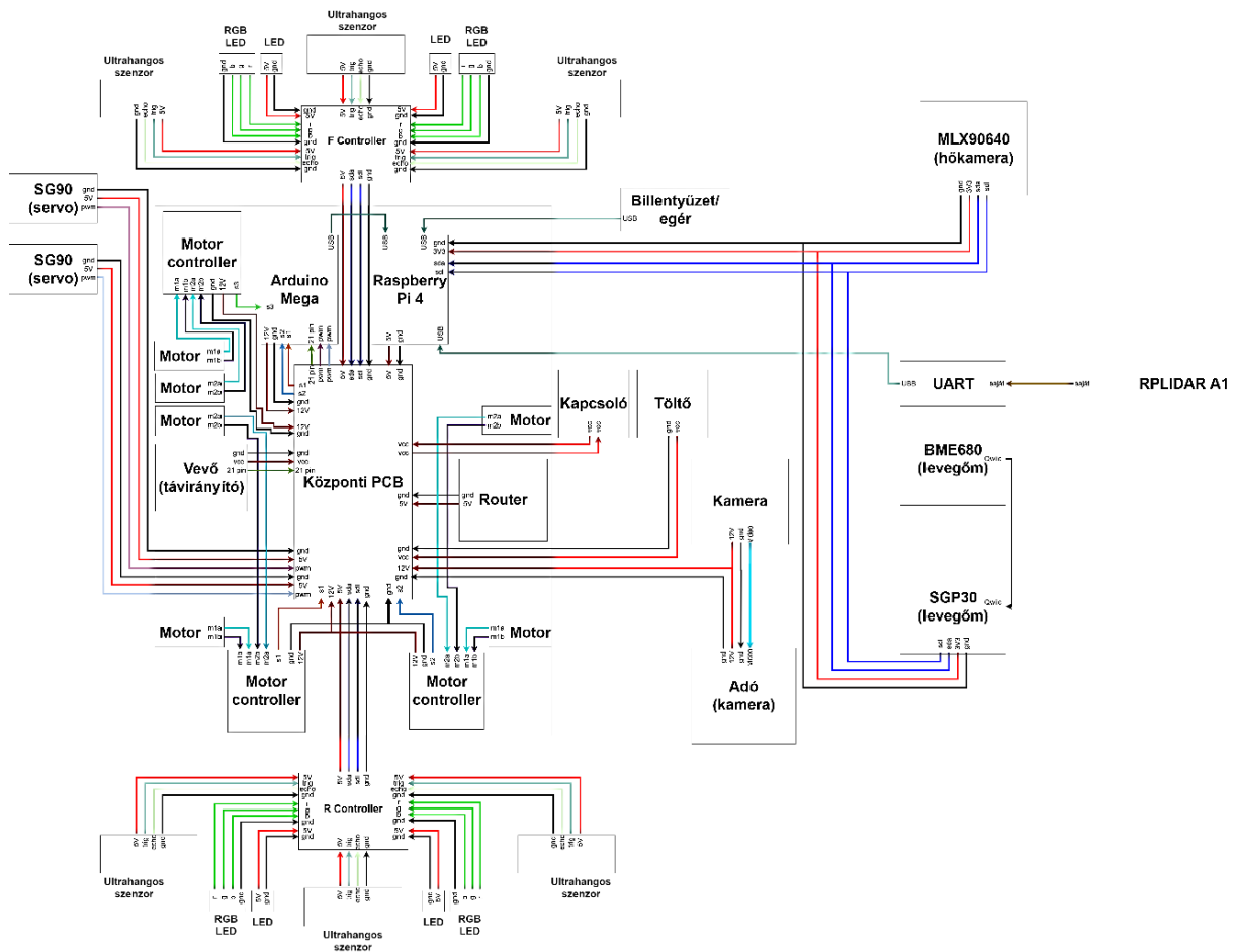
7. ábra: Elektronikai megvalósítás 7
