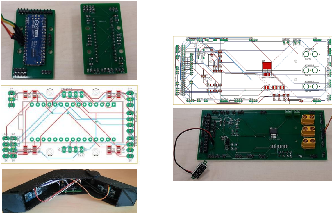
8. ábra: Lőkhárító NYÁK-ok (balra), központi NYÁK jobbra 8
