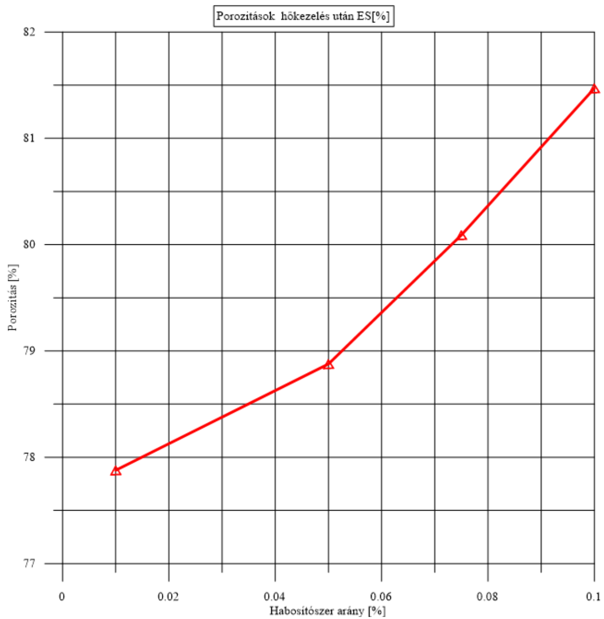
5. ábra Porozitás értékek tojáshéj tartalom esetén hőkezelés után
