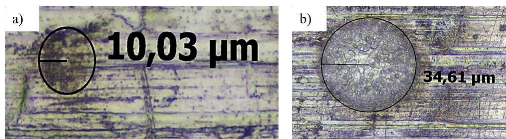
23. ábra: a fs-lézer nyaláb behatásainak vizsgálata a) 10 MHz, P = 10\% b = 3 ; b) 10 MHz, P = 90\% b = 3
