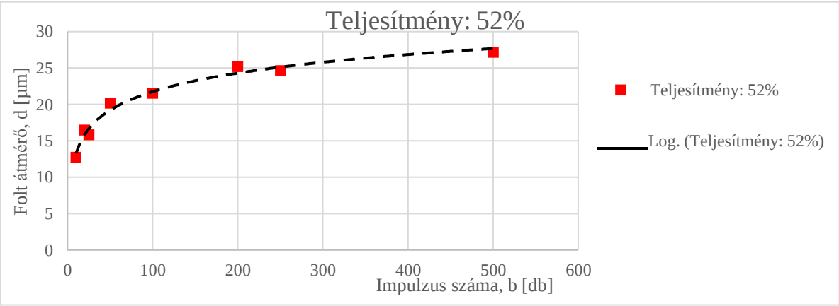
50. ábra: hatásfolt átmérő az impulzus szám függvényében 52% teljesítményen
