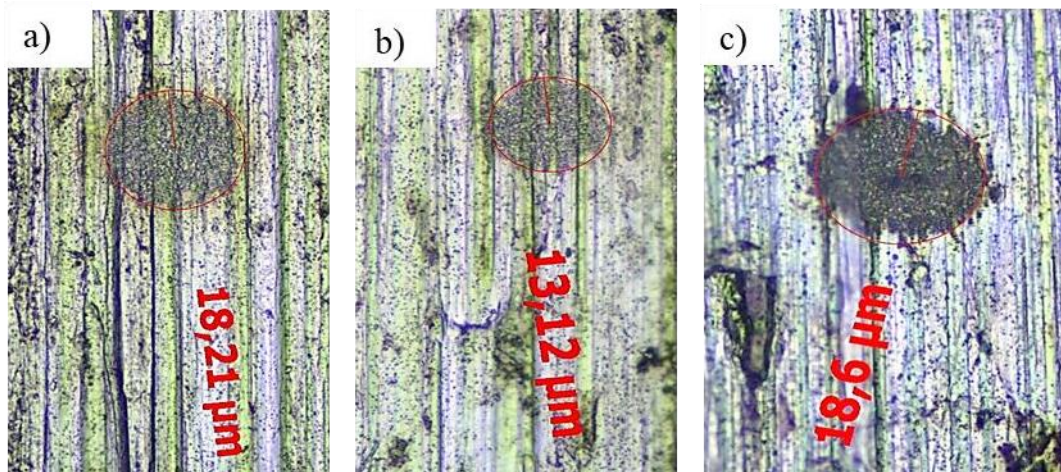
22. ábra: a fs-lézer nyaláb behatásainak vizsgálata a) 10 MHz, P = 52,5\% b = 50 ; b) 10 MHz, P = 55\% b = 20 , c) 10 MHz, P = 55\% b = 50
