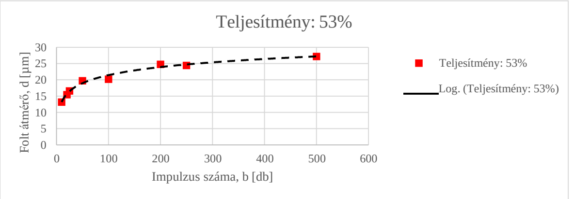
51. ábra: hatásfolt átmérő az impulzus szám függvényében 53% teljesítményen
