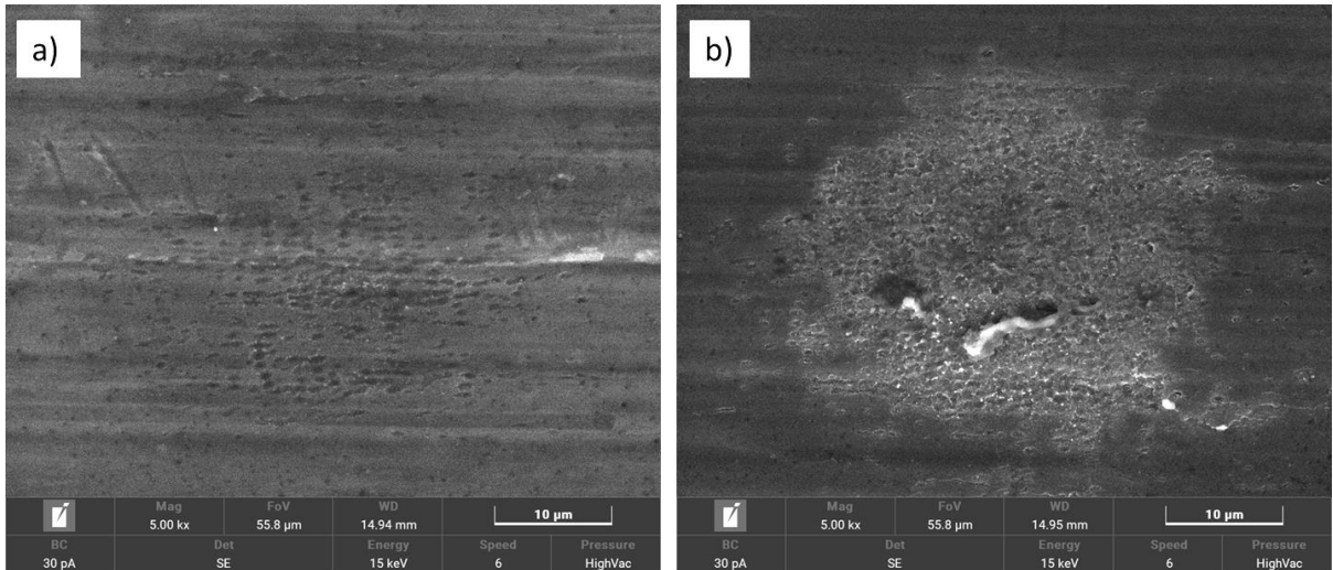
44. ábra: SEM felvétel 25 ismétlés szám mellett a) teljesítmény: 15%; b) teljesítmény: 90%
