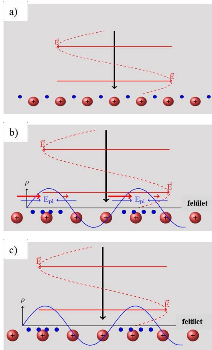
9. ábra: LIPSS keletkezése felületi plazmon interferencia magyarázatával [7]
