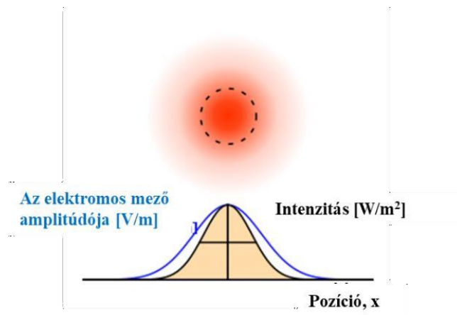
3. ábra: Lézerfókusz intenzitás eloszlása [2]
