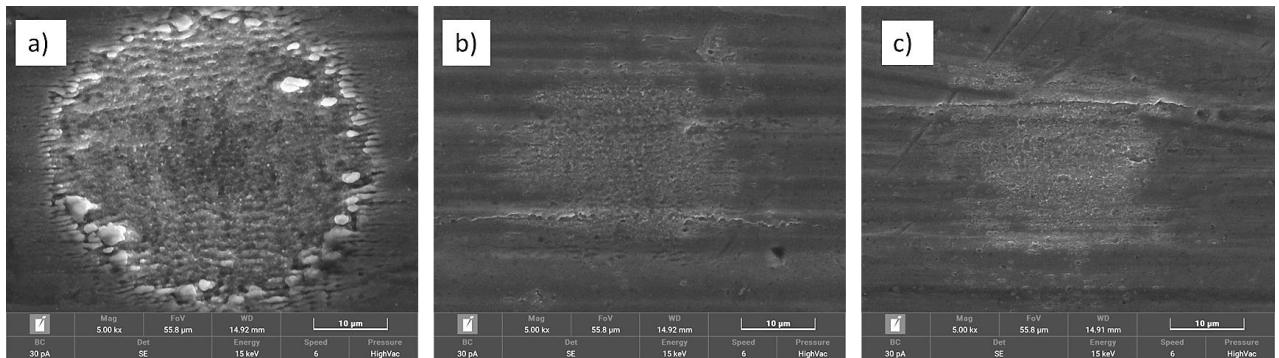
45. ábra: SEM felvétel 50% teljesítmény mellett: a) b=500 ; b) b=10 ; c) b=20
