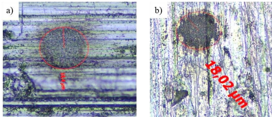
17. ábra: a fs-lézernyaláb behatásainak vizsgálata a) 330 kHz, P = 12,5\% b= 20;
