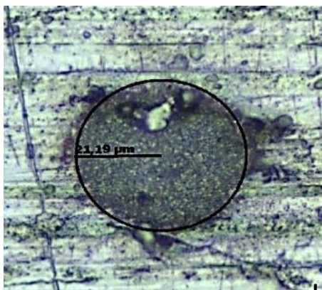
35. ábra: a fs-lézernyaláb behatásainak vizsgálata teljesítmény: 48,5%
