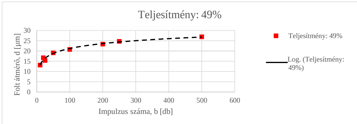
47. ábra: hatásfolt átmérő az impulzus szám függvényében 49% teljesítményen
