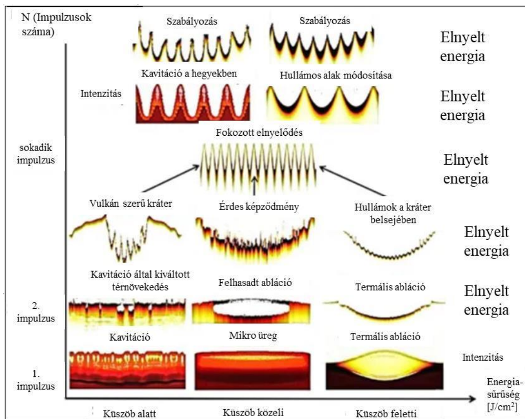
55. ábra: A lézeres megmunkálás során bekövetkező folyamatok [6]
