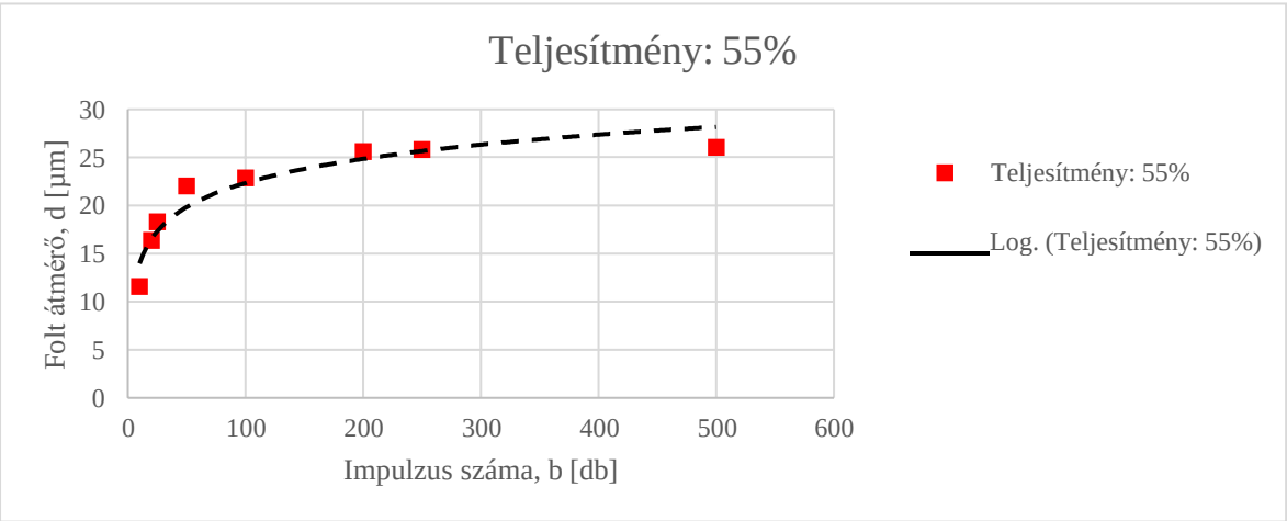
54. ábra: hatásfolt átmérő az impulzus szám függvényében 55% teljesítményen
