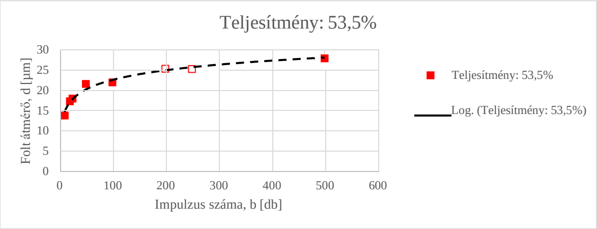
52. ábra: hatásfolt átmérő az impulzus szám függvényében 53,5% teljesítményen
