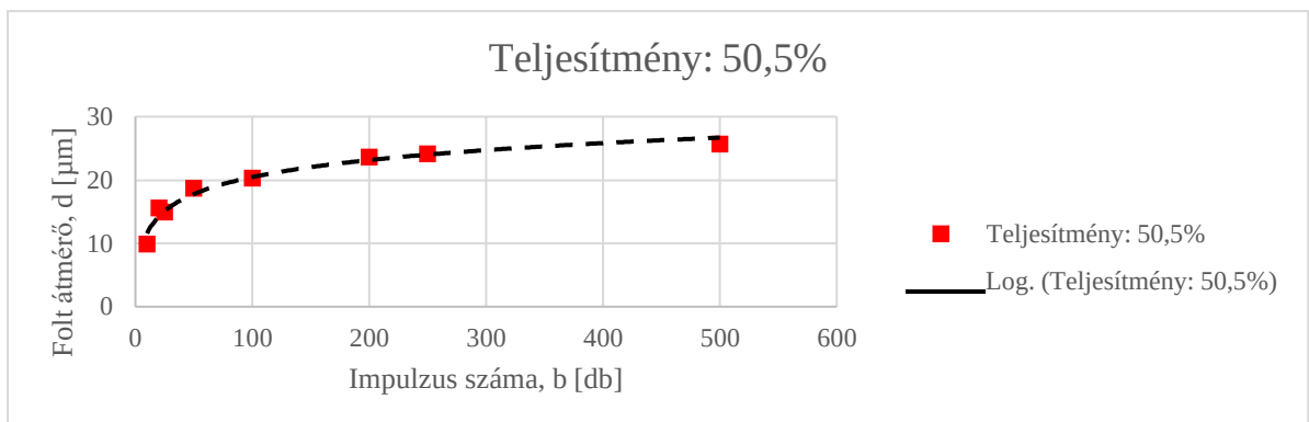
48. ábra: hatásfolt átmérő az impulzus szám függvényében 50,5% teljesítményen
