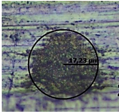
40. ábra: a fs-lézernyaláb behatásainak vizsgálata teljesítmény: 53%
