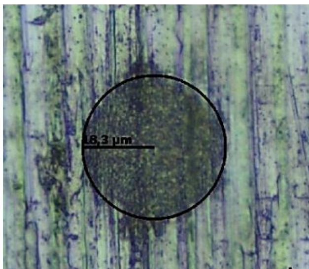
43. ábra: a fs-lézernyaláb behatásainak vizsgálata teljesítmény: 55%
