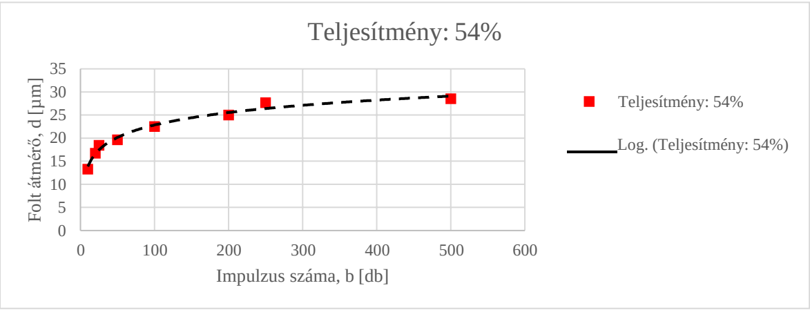
53. ábra: hatásfolt átmérő az impulzus szám függvényében 54% teljesítményen
