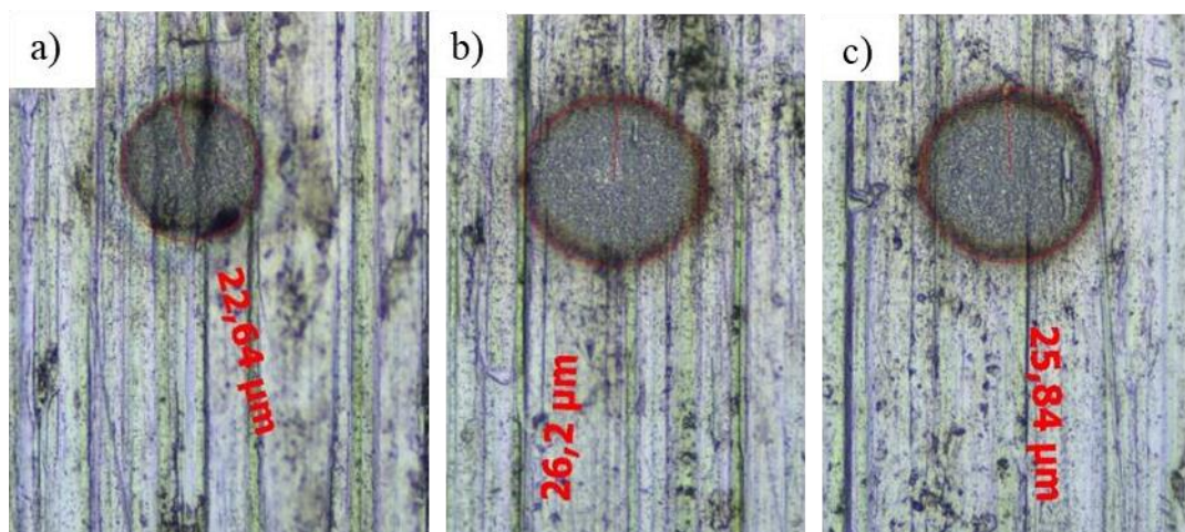
18. ábra: a fs-lézernyaláb behatásainak vizsgálata a) 330 kHz, P = 15\% b= 50; b) 330
