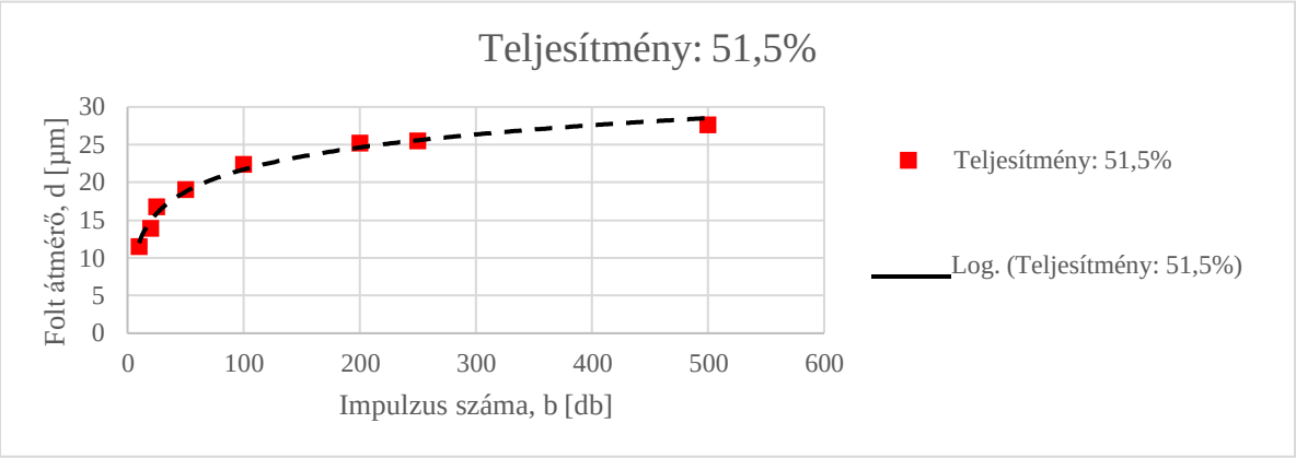
49. ábra: hatásfolt átmérő az impulzus szám függvényében 51,5% teljesítményen
