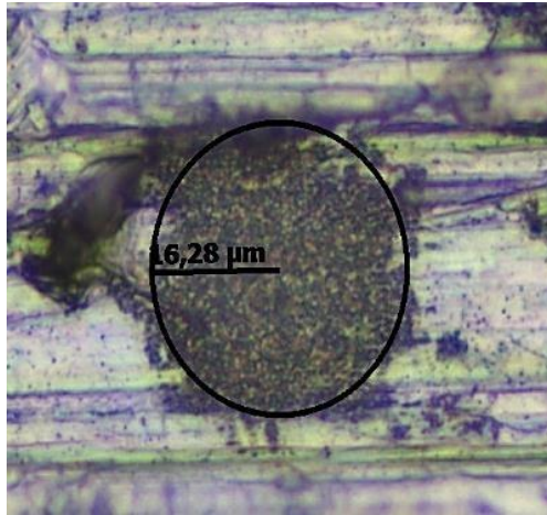
26. ábra: a fs-lézernyaláb behatásainak vizsgálata teljesítmény: 45%, impulzusszám: 500
