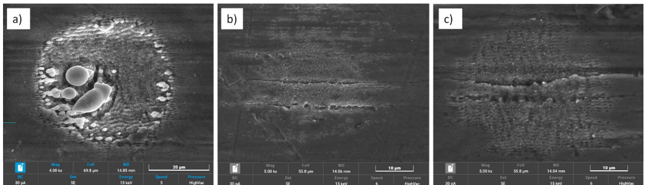
46. ábra: SEM felvétel 55% teljesítmény mellett: a) b=500 ; b) b=10 ; c) b=50
