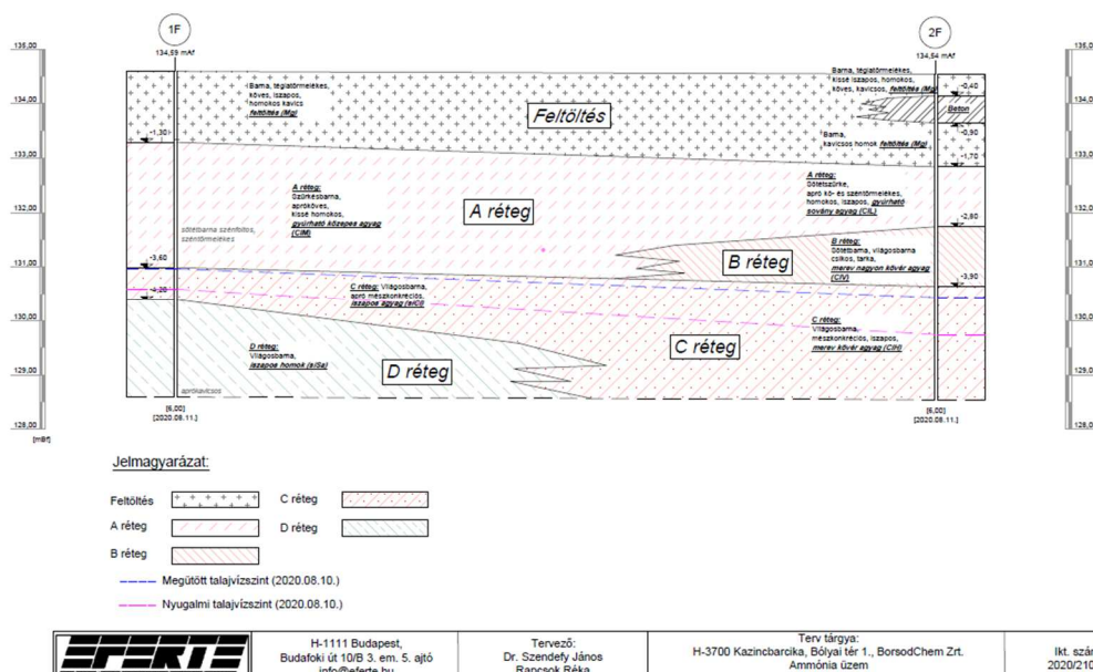
V.2.1.kép. Talajvizsgálati jelentés rétegszelvénye
