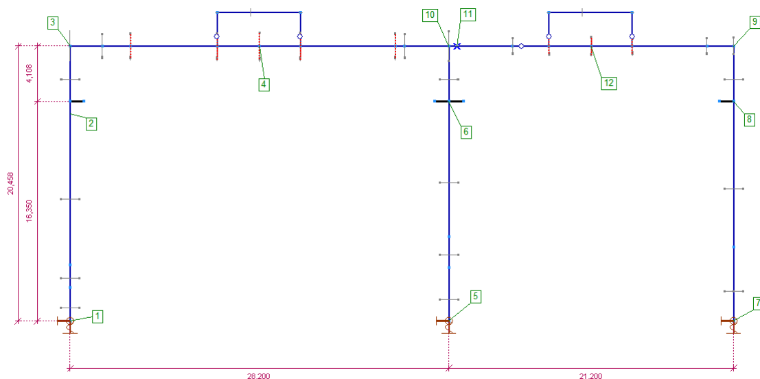
V.1.1.kép. Keretszerkezet statikai váza és jellemző csomópontjai
