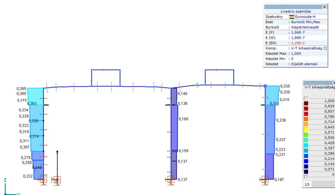
VII.1.12.kép. Keretszerket kihasználtsága V-T igénybevételekkel szemben
