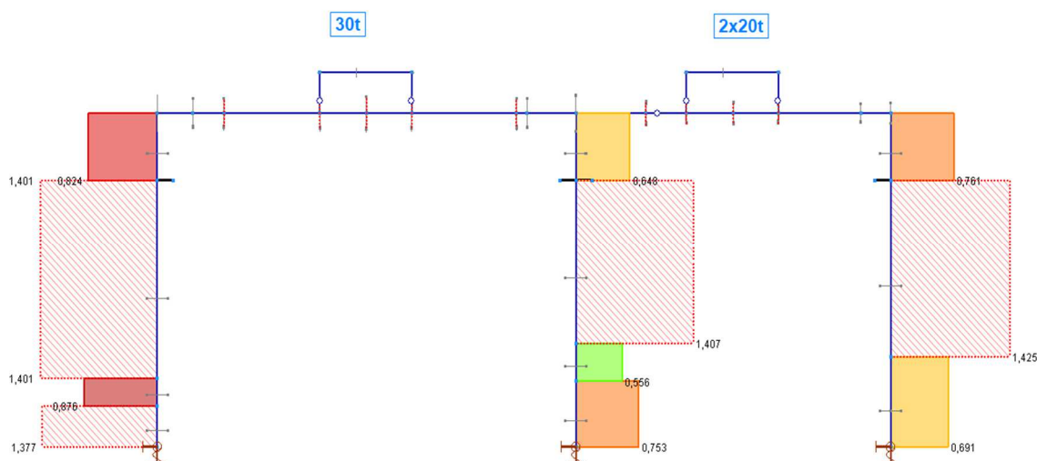
V.1.2.kép. Keretoszlop N-M kihasználtságai
