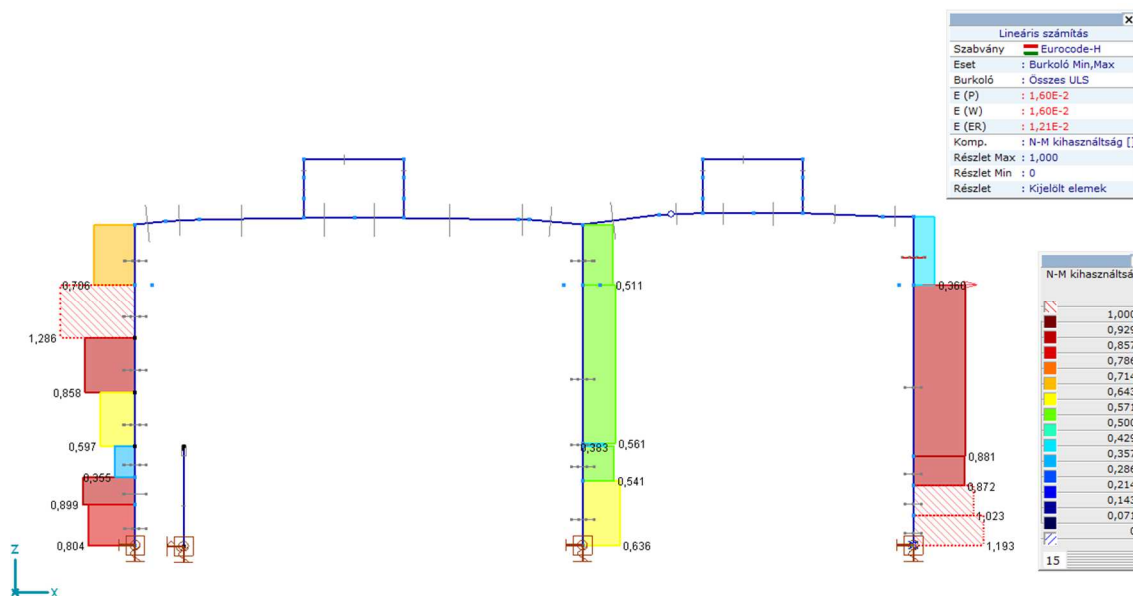
VII.1.3.kép. Keretszerket kihasználtsága N-M igénybevételekkel szemben
