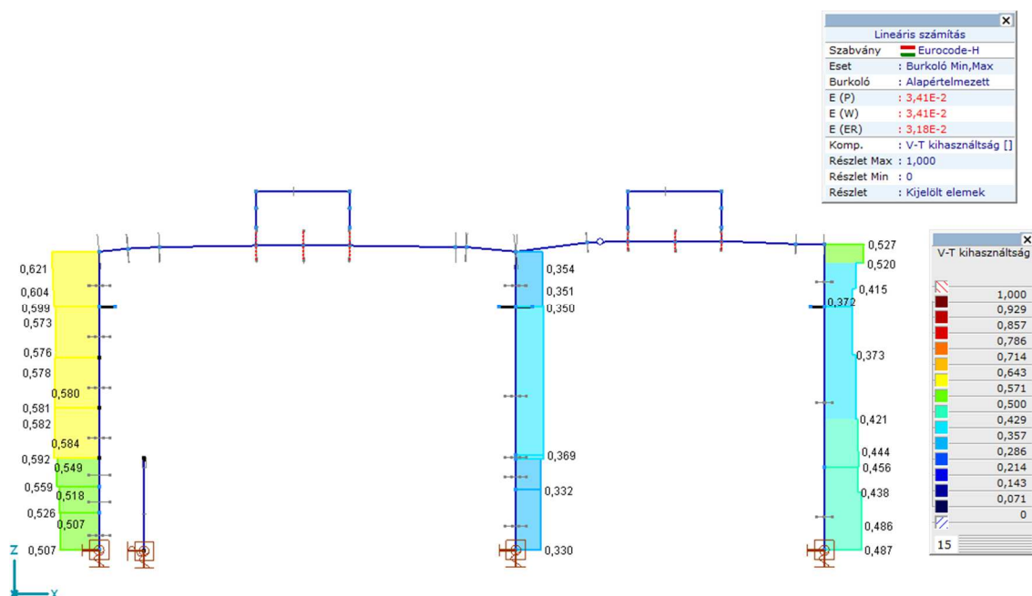
VII.1.2.kép. Keretszerket kihasználtsága V-T igénybevételekkel szemben
