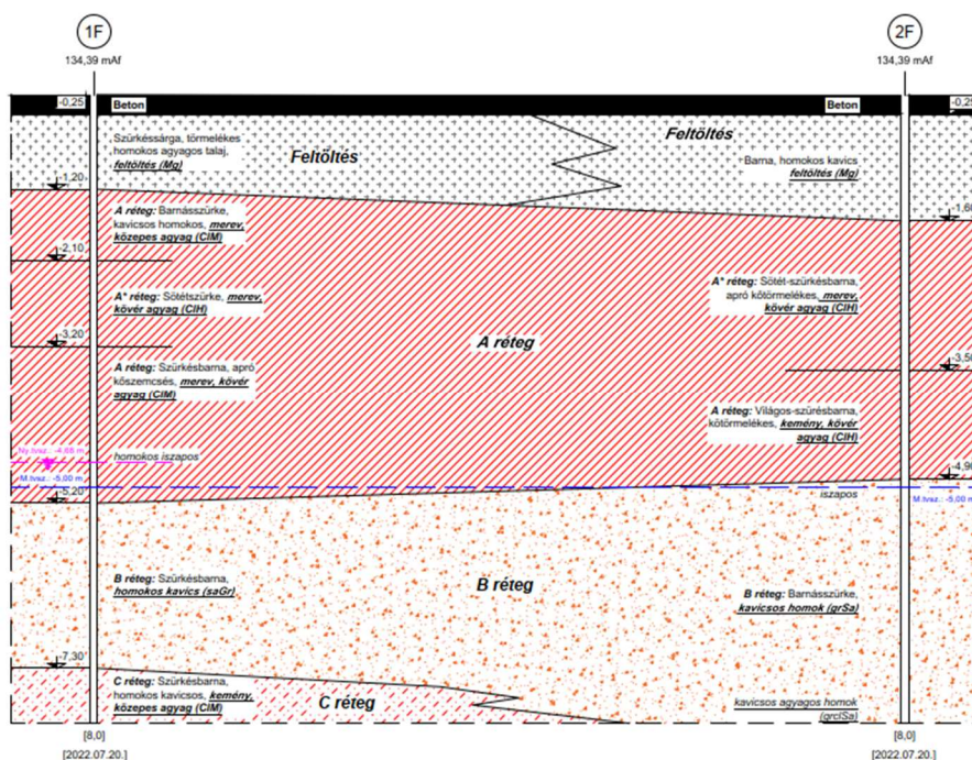
VII.3.1.kép. Talajvizsgálati jelentés rétegszelvénye
