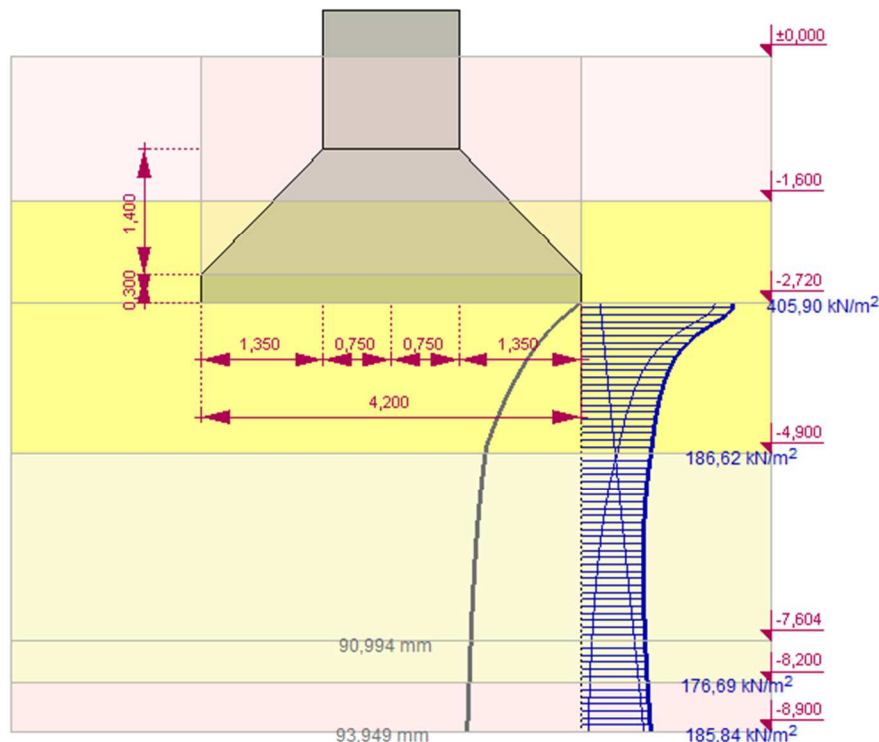
VII.3.3.kép. Becsült alaptest teherbírás középső ker.oszl. alatt
