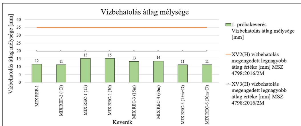
4.22. ábra: 1. próbakeverés: Vízárósági vizsgálat során mért átlagos vízbehatolási mélység [saját vizsgálat alapján]
