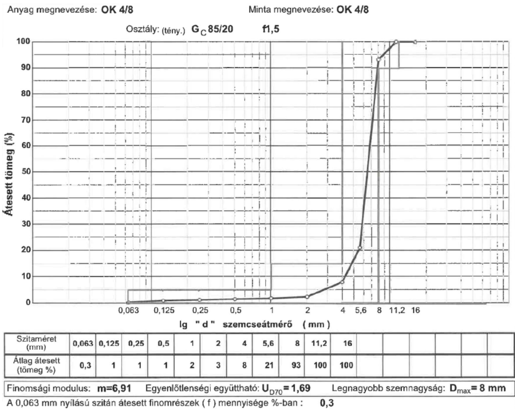
10. sz. melléklet: OK 4/8 Vizsgálati jegyzőkönyv; Szitavizsgálat MSZ EN 933-1:2012 szerint
