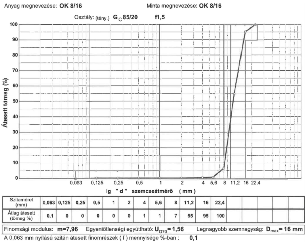
11. sz. melléklet: OK 8/16 Vizsgálati jegyzőkönyv; Szitavizsgálat MSZ EN 933-1:2012 szerint
