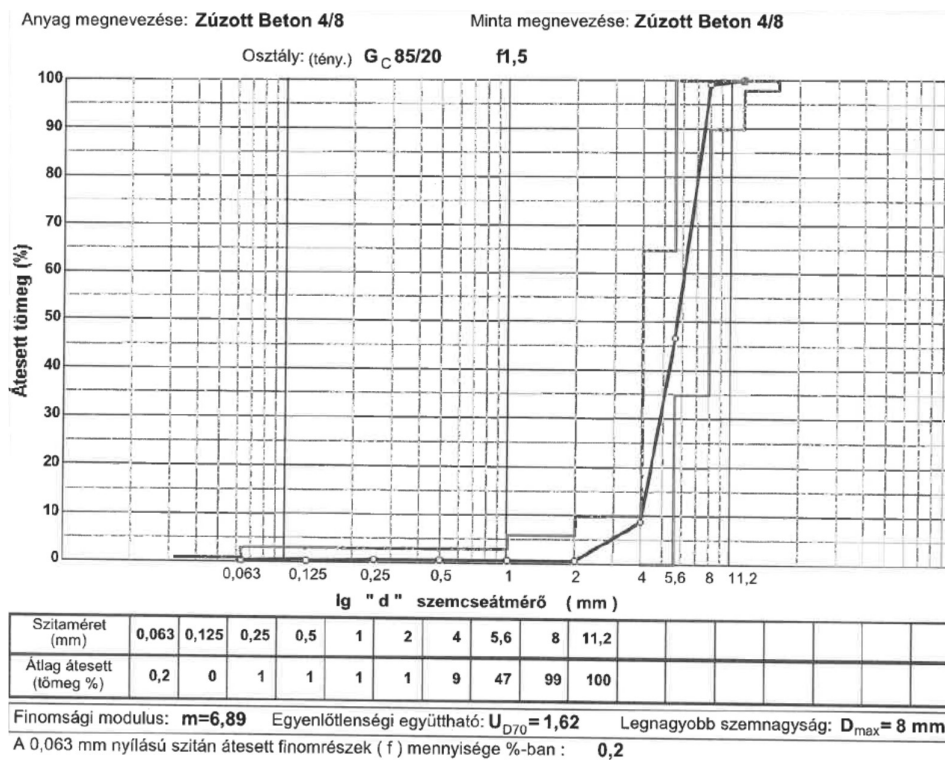
4.11. ábra: Zúzott adalékanyag 4/8 szemmegoszlási görbéje MSZ EN 933-1:2012 [saját
