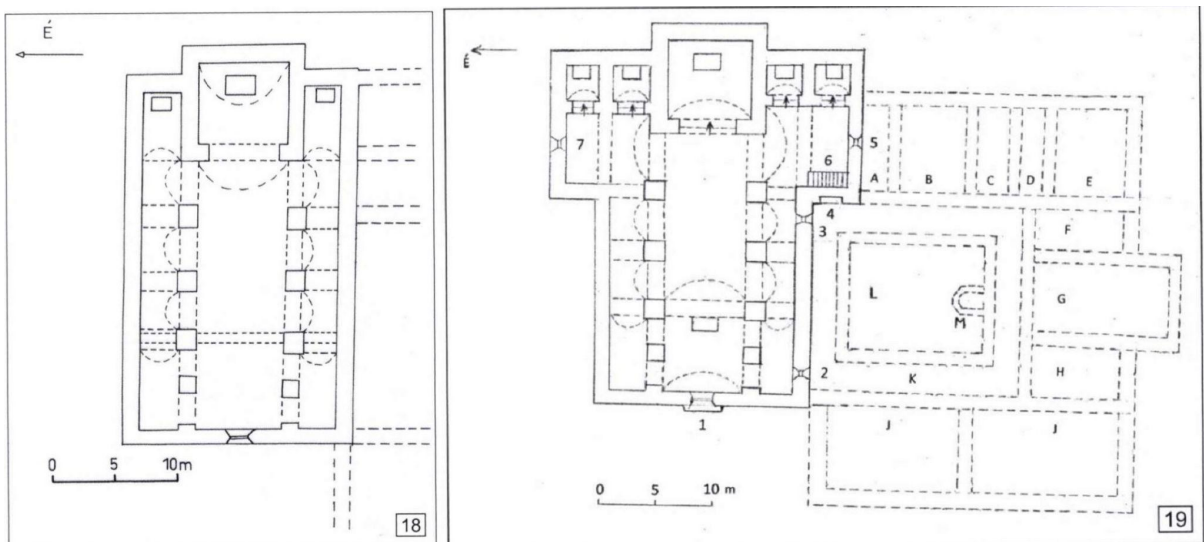
3. A cikádori templom első és második - feltételezett - építési periódusának alaprajza, 2001
