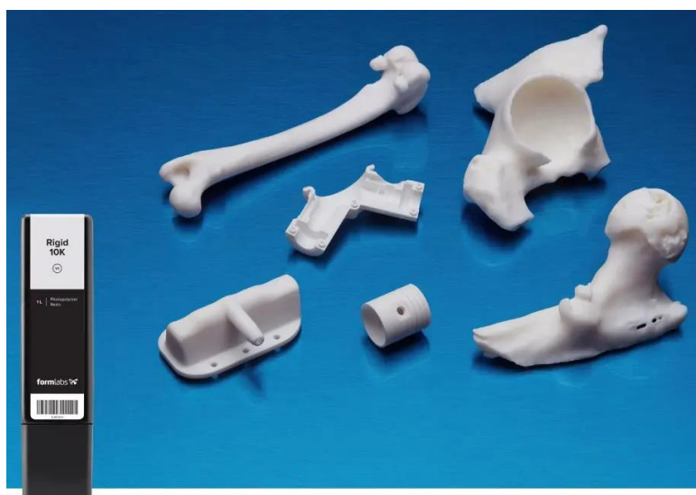
30. ábra: Formlabs Rigid 10k gyantából készített 3D modellek 47
