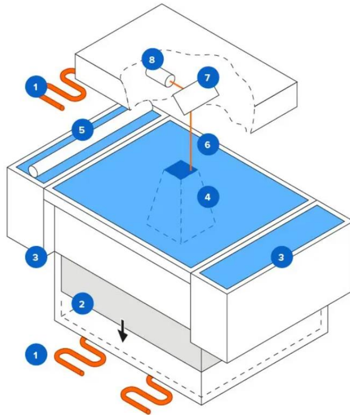
5. ábra: SLS nyomtató ábrája 14
