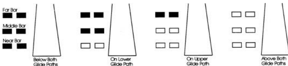
8. Ábra- Visual Approach Slope Indicator működésének ábrázolása.
