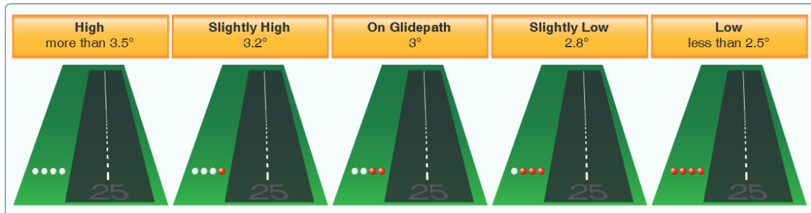
7. Ábra- Precision Approach Path Indicator működésének ábrázolása.
