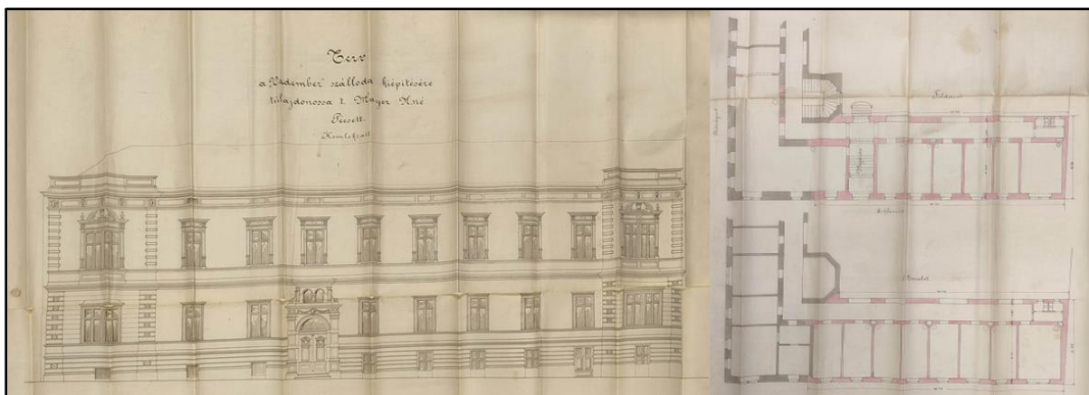
17. kép: A Vadember Szálloda 1886-os eredeti homlokzati terve (bal) és alaprajza (jobb)
