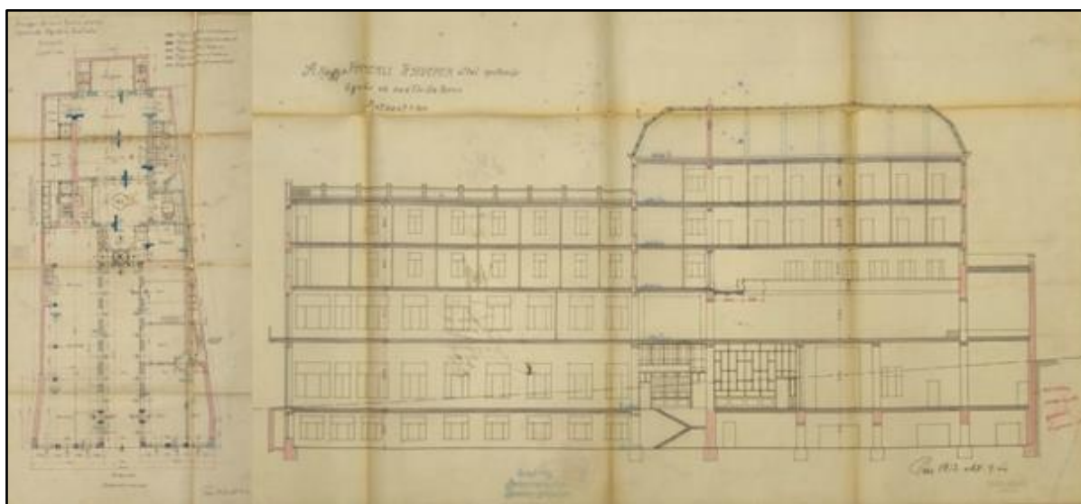
23. kép: A Pannonia Szálló földszinti alaprajza (bal) és hosszmetseti képe (jobb) az 1912-es tervekből
