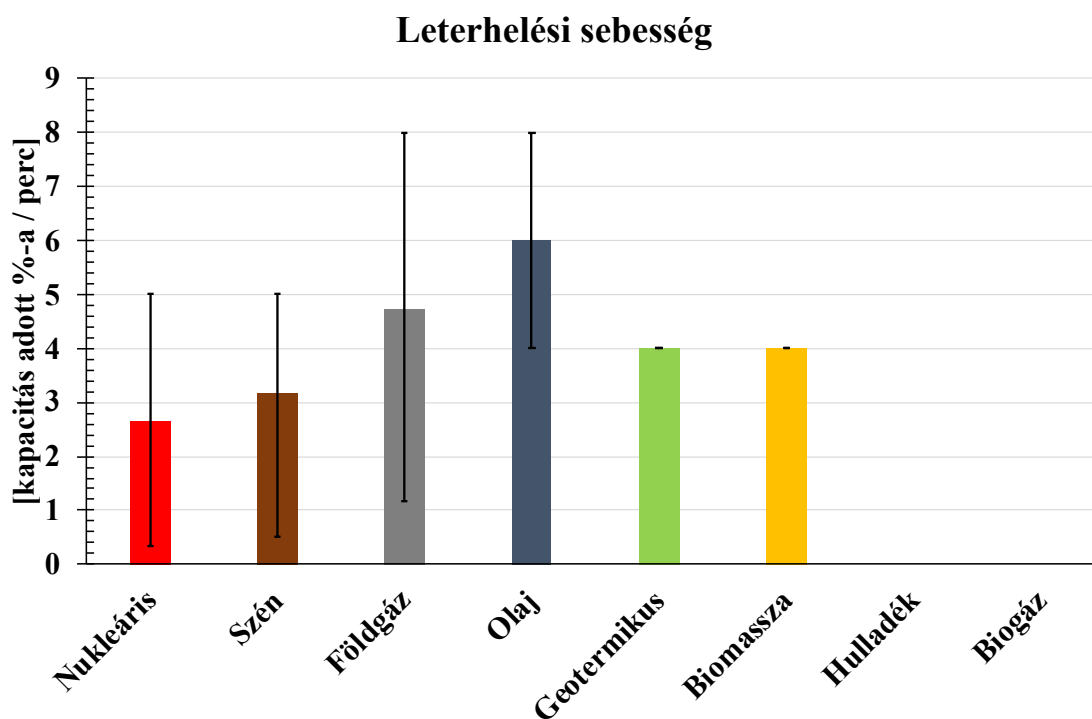
37. ábra Az erőművek leterhelési sebesség PLEXOS inputja az irodalomkutatás alapján (adatok forrása [32, 33, 38], saját ábrázolás)
