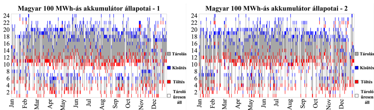
17. ábra A magyar 100 MWh-ás akkumulátor állapotainak órás bontása az 1. scenárióban (bal) és a 2. scenárióban (jobb) 2030-ban
