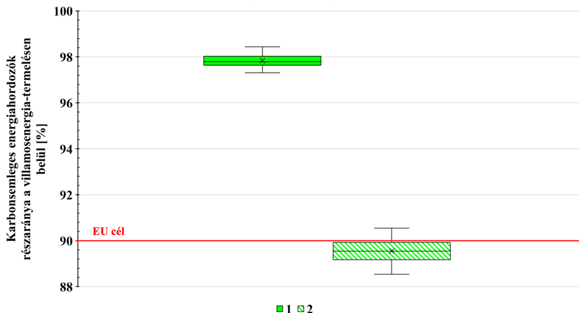
14. ábra Magyarország 2030-as karbonsemleges villamosenergia-termelésének ingadozására irányuló érzékenységi vizsgálat (nap- és szél erőművek órás kihasználási tényezője 40 évnyi adat alapján)
