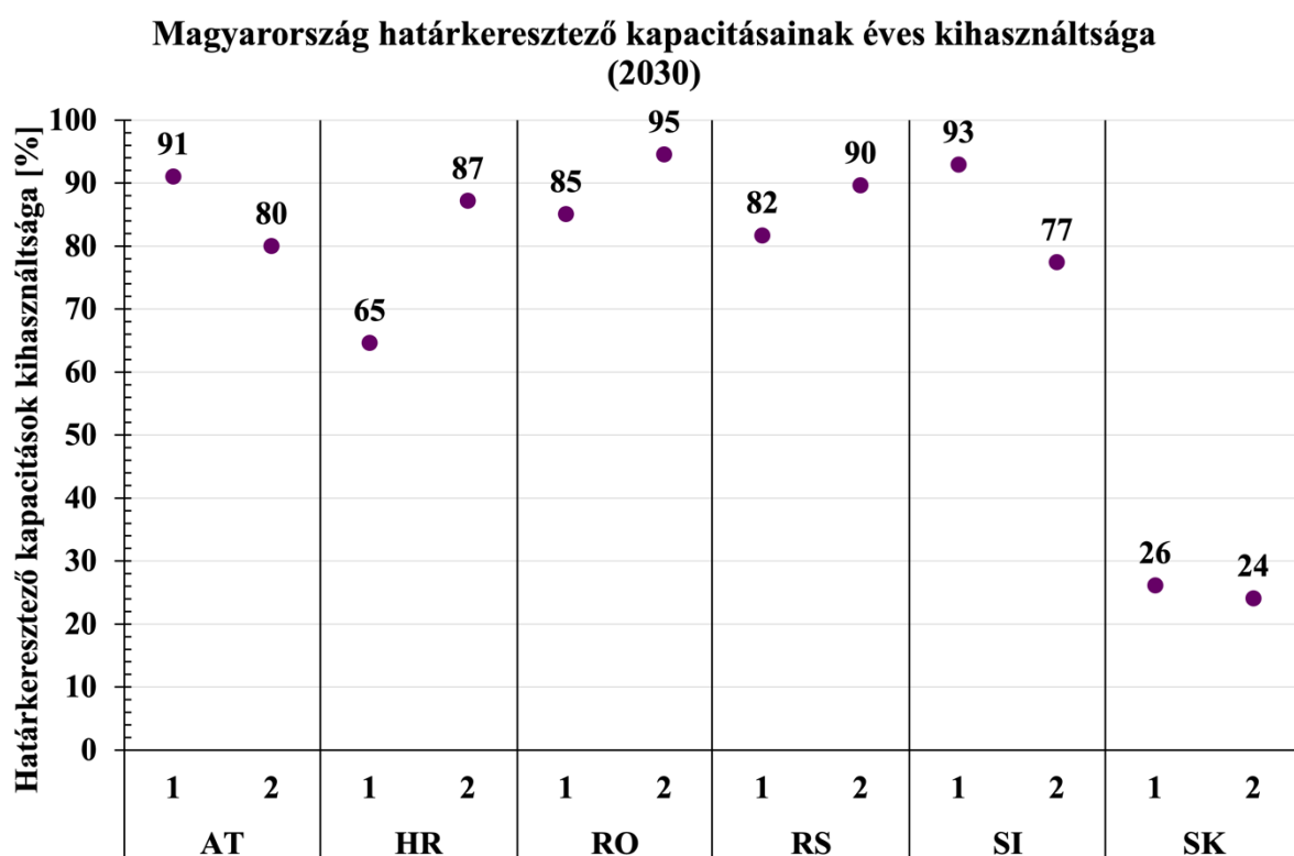
31. ábra A magyar határkeresztező kapacitások éves kihasználtsága a két scenárióban 2030-ban
