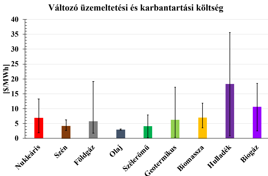
34. ábra Az erőművek változó üzemeltetési és karbantartási költség PLEXOS inputja az irodalomkutatás alapján (adatok forrása [25, 32, 36–38, 41, 42] saját ábrázolás)
