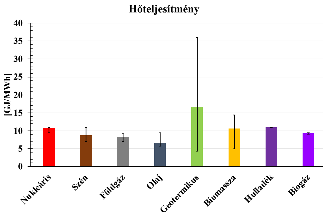
33. ábra A hőteljesítmény PLEXOS inputja az irodalomkutatás alapján (adatok forrása [25, 32, 34–40], saját ábrázolás)
