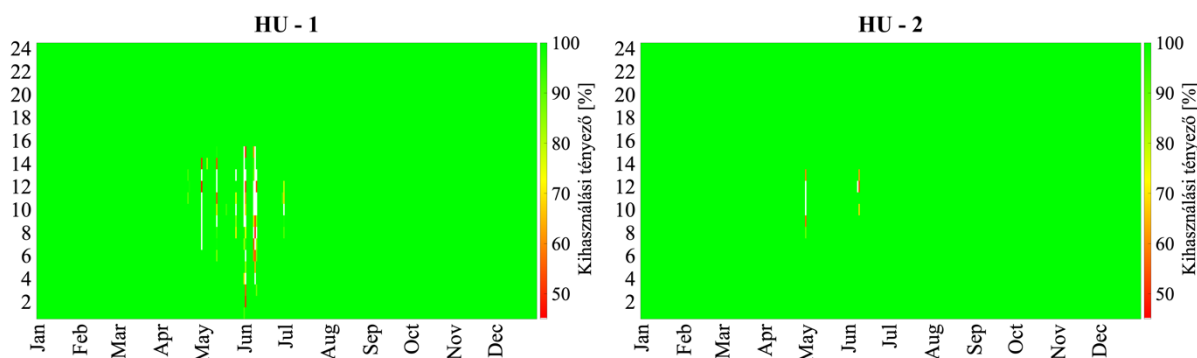
30. ábra A magyar atomerőmű flotta teljesítménykihasználási-tényezőjének órás lefutása az 1. scenárióban (balra), és a 2. scenárióban (jobbra)
