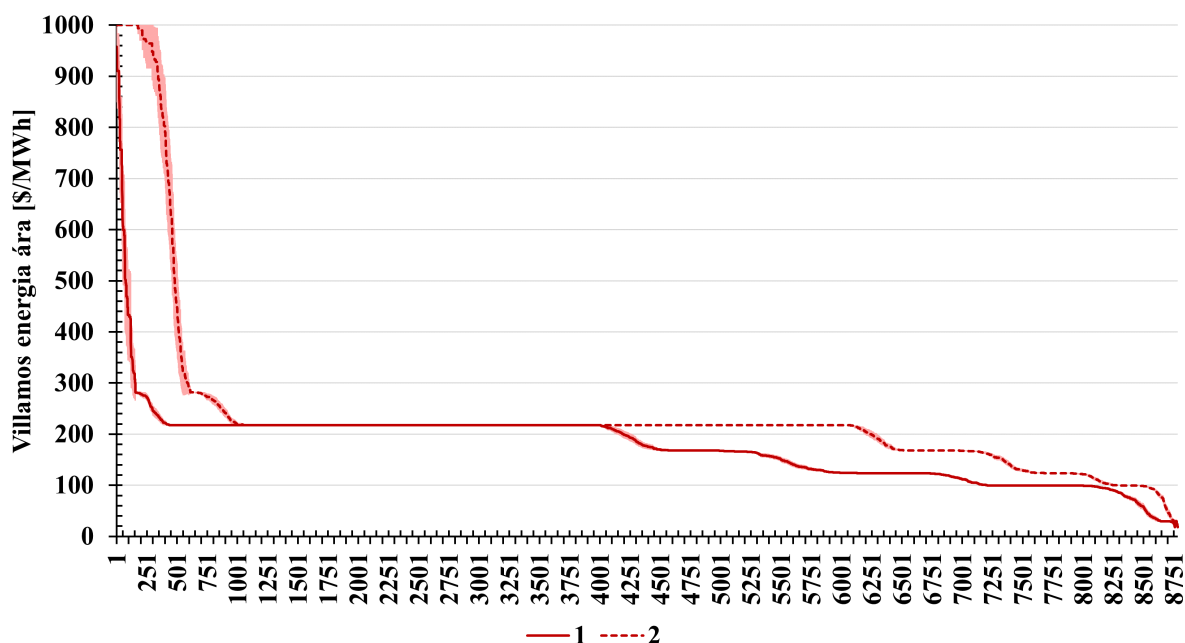
25. ábra A magyar villamosenergia-piacon kialakuló villamos energia átlagos árának tartamdiagramja az 1. scenárióban (folytonos vonal) és a 2. scenárióban (szaggatott vonal) 2030-ban, feltüntetve az órás értékek 95 %-os konfidenciaszinthez tartozó bizonytalansági sávját is (nap- és szélerőművek órás kihasználási tényezője 40 évnyi adat alapján)
