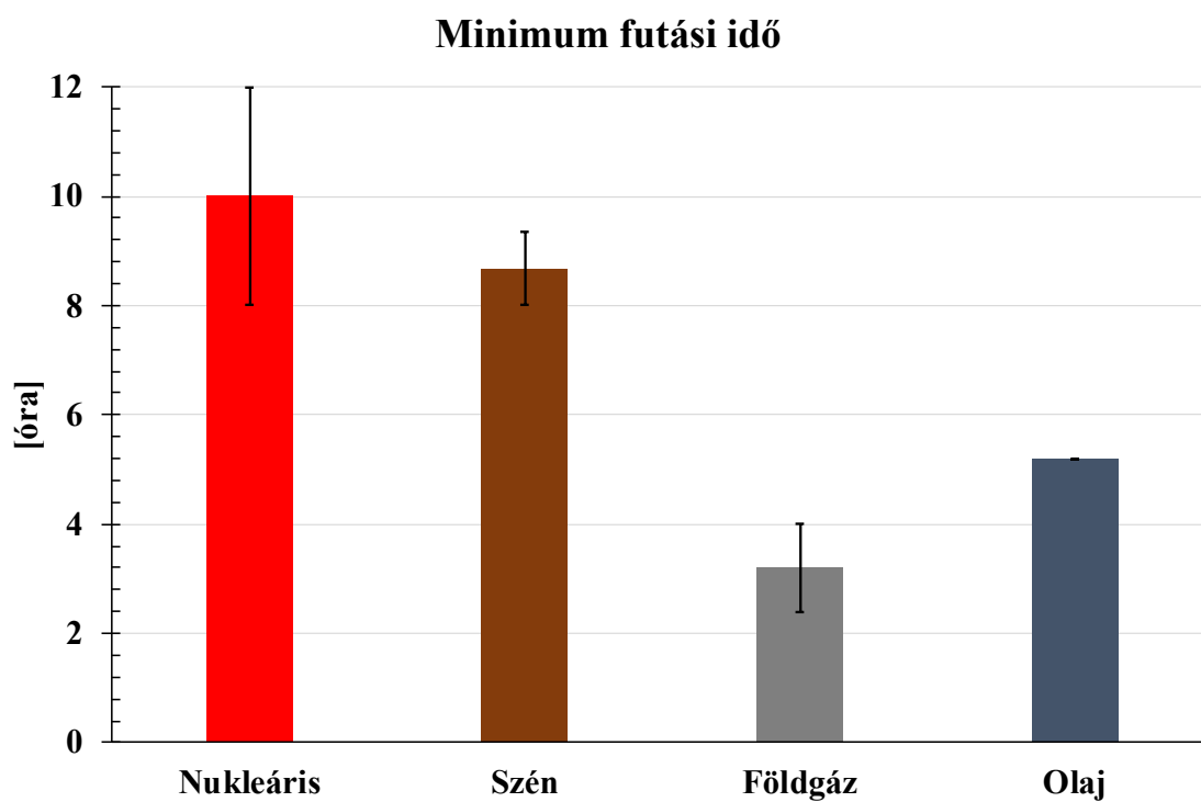
38. ábra Az erőművek minimum futási idő PLEXOS inputja az irodalomkutatás alapján (adatok forrása [32, 38], saját ábrázolás)
