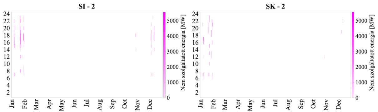
42. ábra A országokban kialakult nem szolgáltatott energia mennyiségének órás lefutása a két szcenárióban 2030-ban
