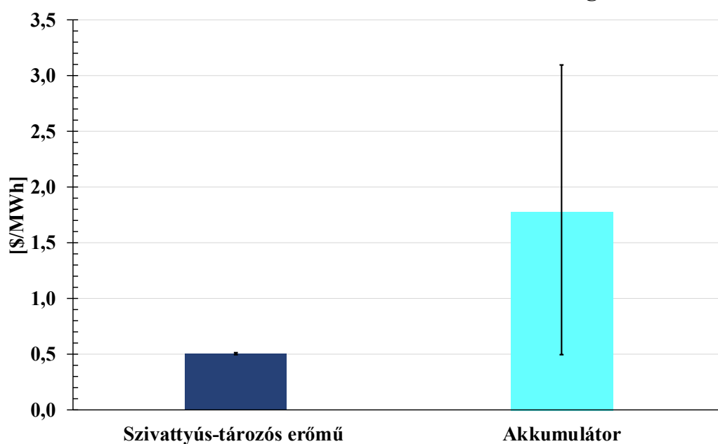
41. ábra A szivattyús-tározós erőművek és az akkumulátoros villamosenergia-tároló egységek változó üzemeltetési és karbantartási költség PLEXOS inputja az irodalomkutatásom alapján (adatok forrása [44, 45, 50, 51, 56, 57], saját ábrázolás)
