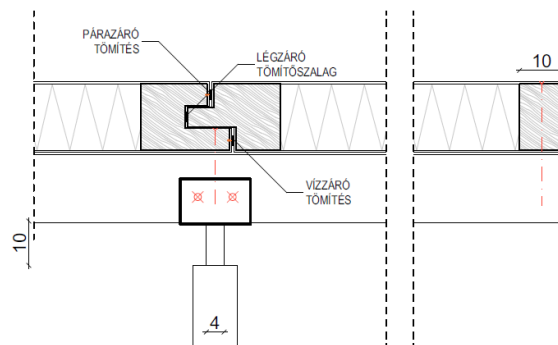
23. ábra: Padló hosszsz metszeti csomópont [saját]
