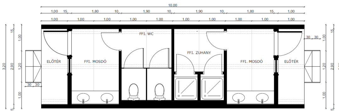
37. ábra: Férfi vizesblokk [saját]
