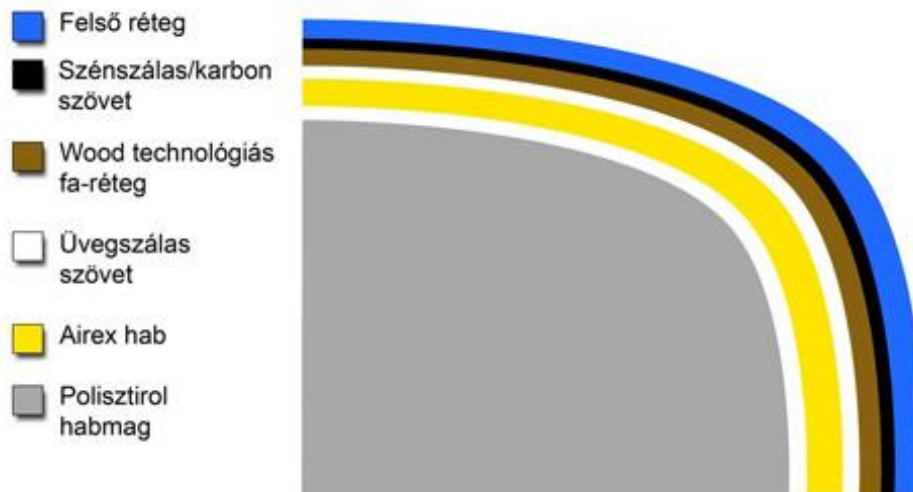
17. ábra: A duroplasztikus szörfdeszka felépítése [18]
