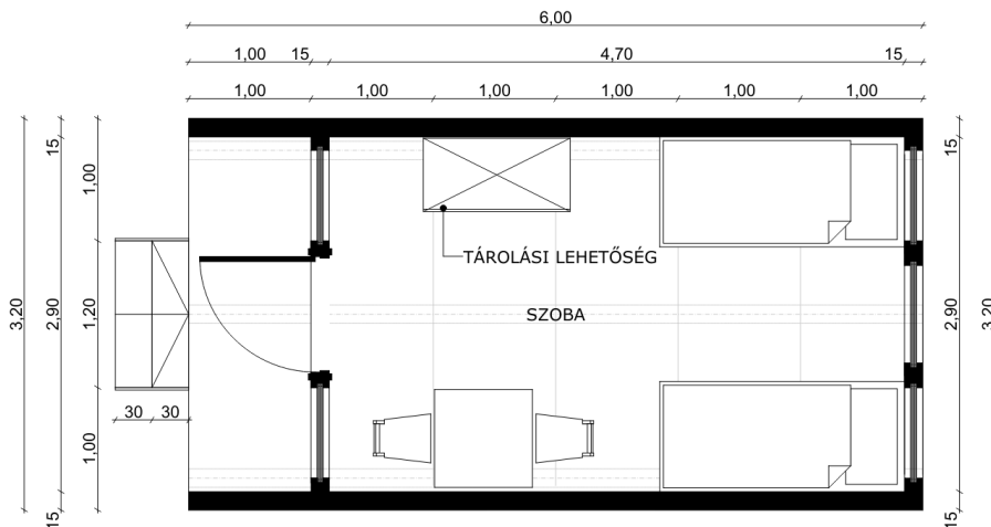
34. ábra: Általános alaprajz 2 főre [saját]
