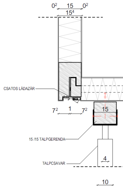
25. ábra: Padló keresztmetszeti csomópont [saját]
