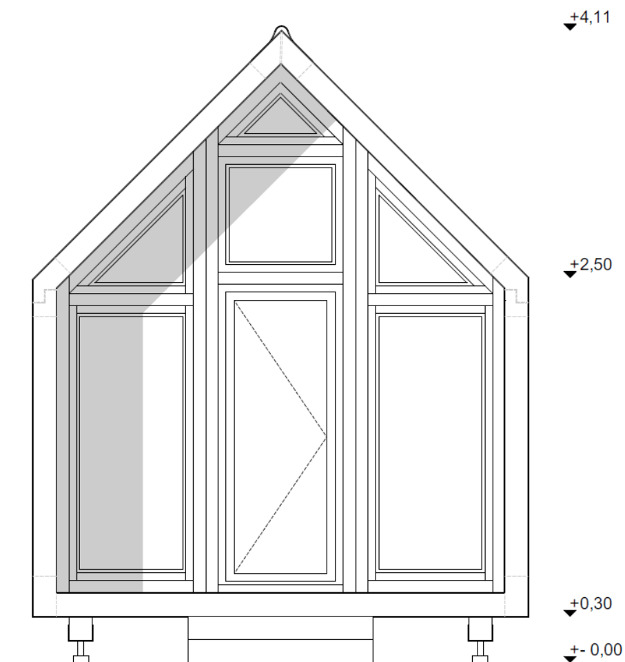
44. Bejárat homlokzat [saját]
