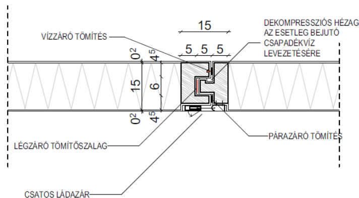
26. ábra: Fal és tető csomópont [saját]
