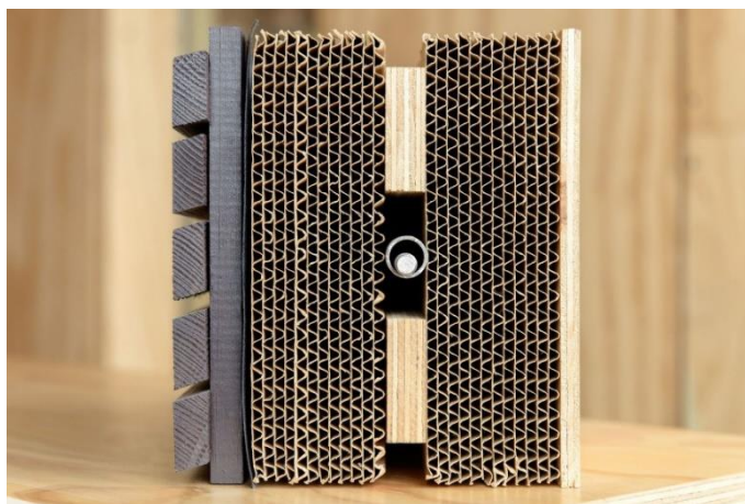
16. ábra: Karton házrendszer [17]
