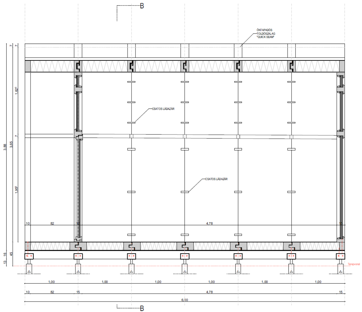
42. ábra: Hosszmetszet [saját]
