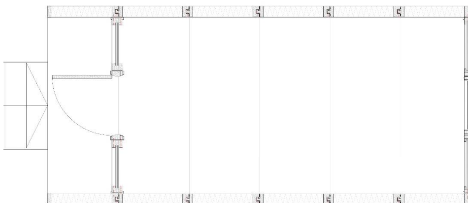
33. ábra: Alaprajz [saját]
