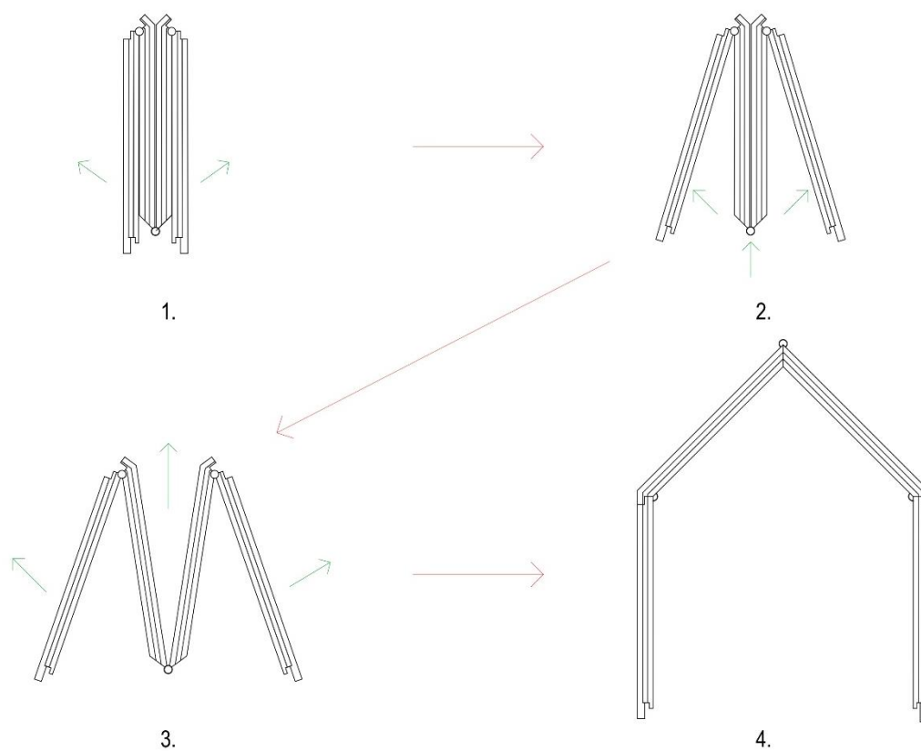
22. ábra: Kihajtás lépései [saját]
