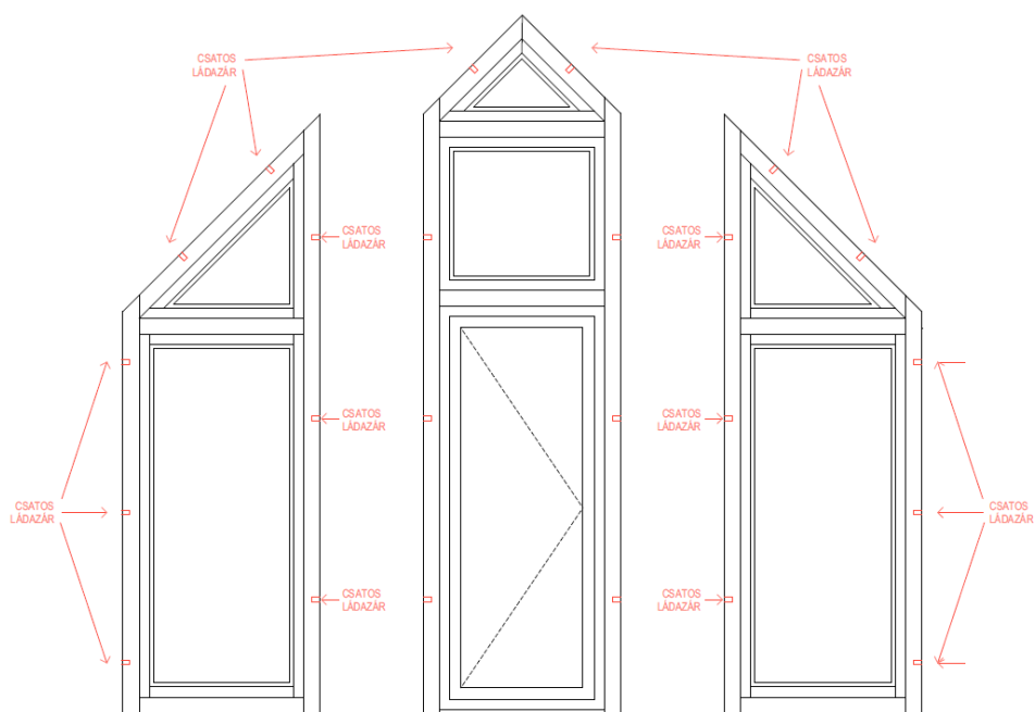
45. Ablakok kialakítása [saját]
