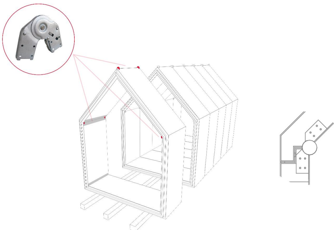
28. ábra: 3D ábra [saját]
