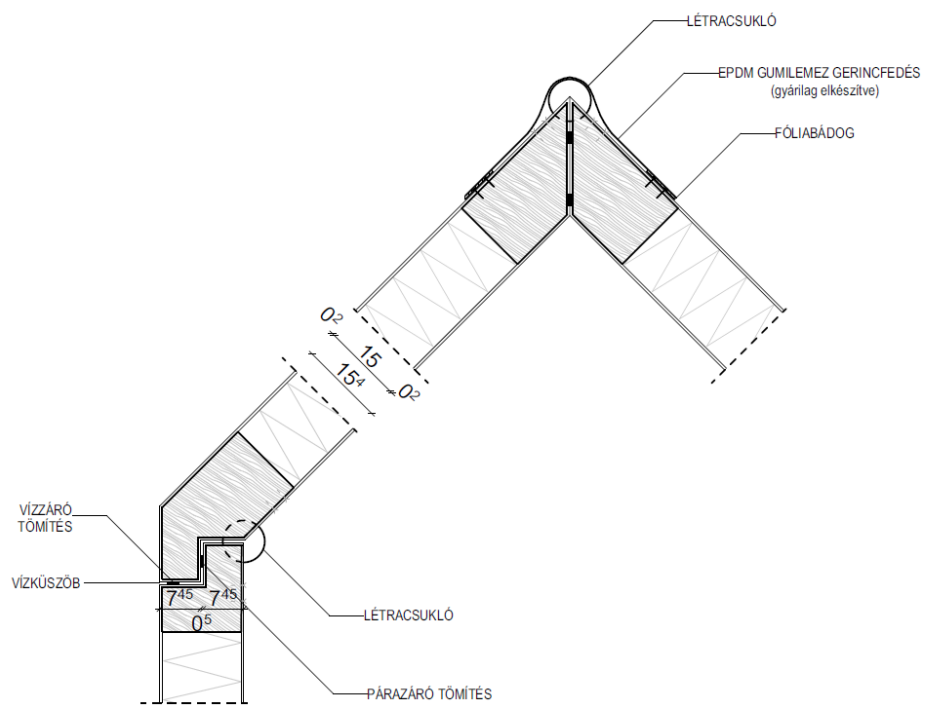
27. ábra: Tető hajlás csomópont [saját]
