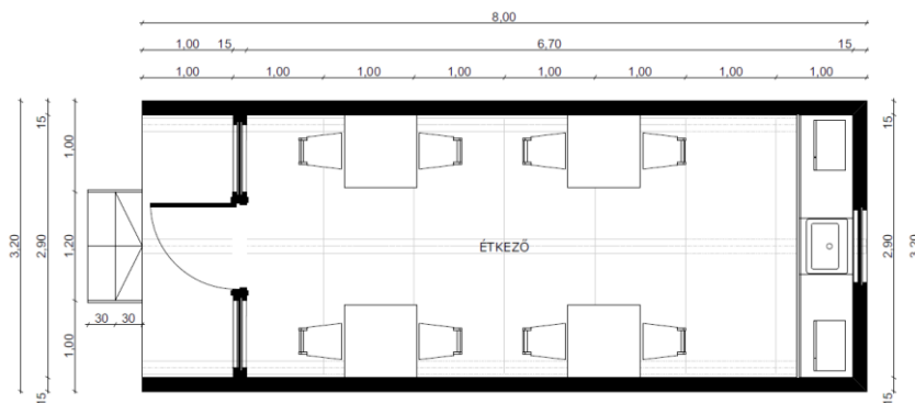
40. ábra: Konyha egység [saját]
