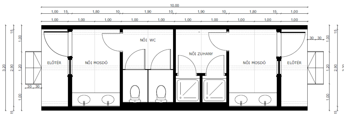
36. ábra: Női vizesblokk [saját]
