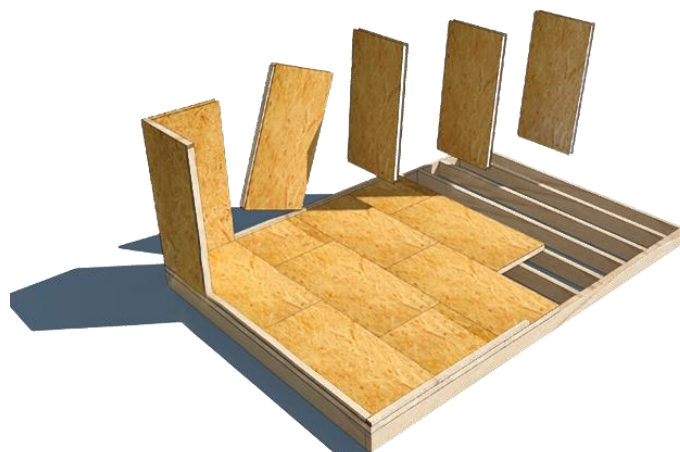
15. ábra: SIP rendszer [16]
