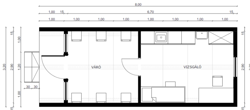
39. ábra: Elsősegély egység [saját]
