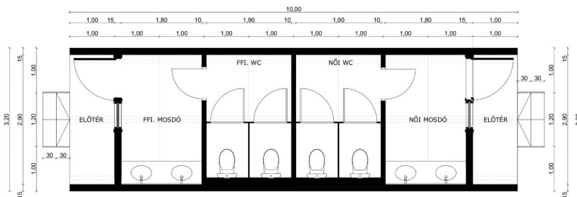
38. ábra: Férfi-Női vizesblokk [saját]
