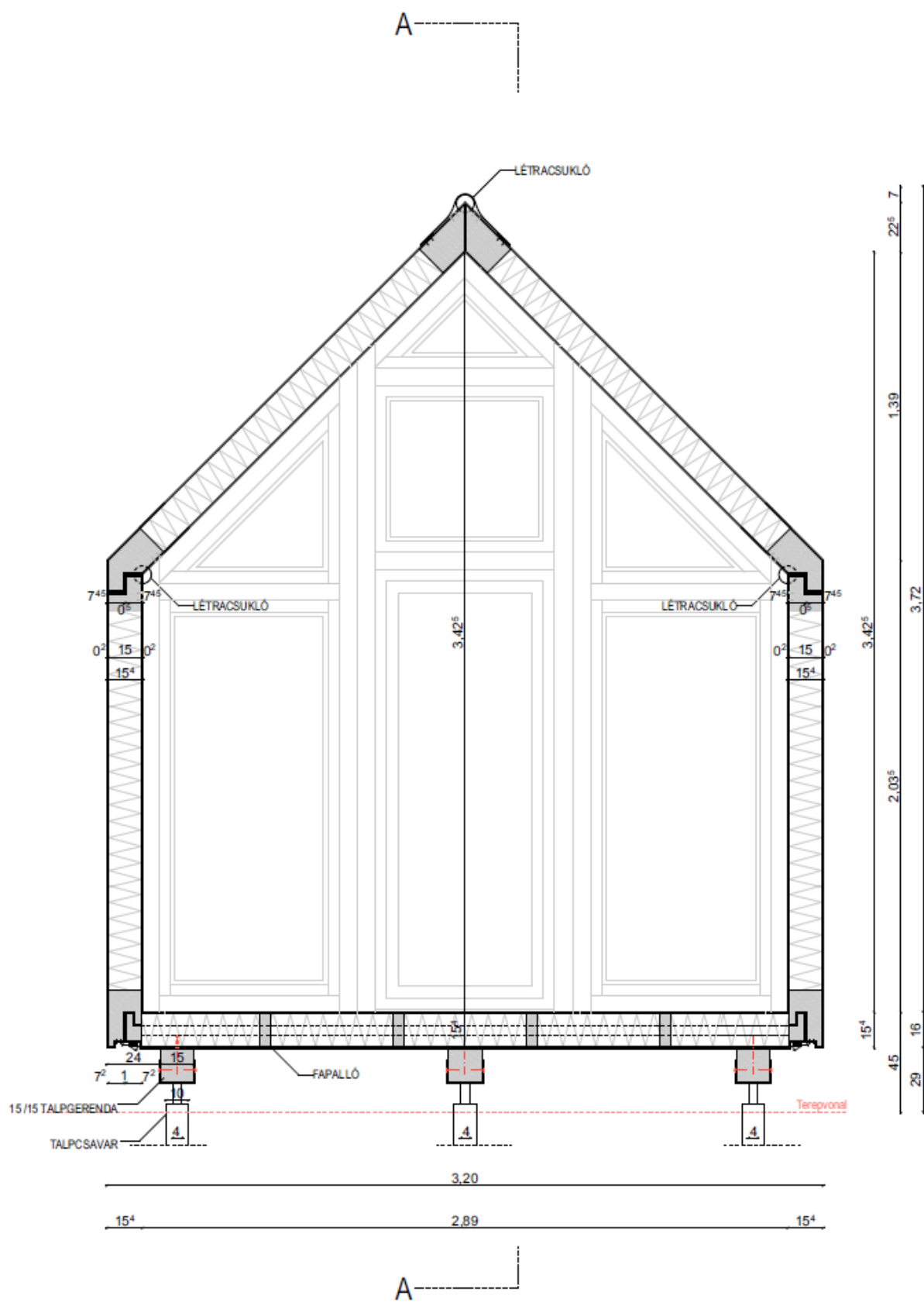
41. ábra: Keresztmetszet [saját]
