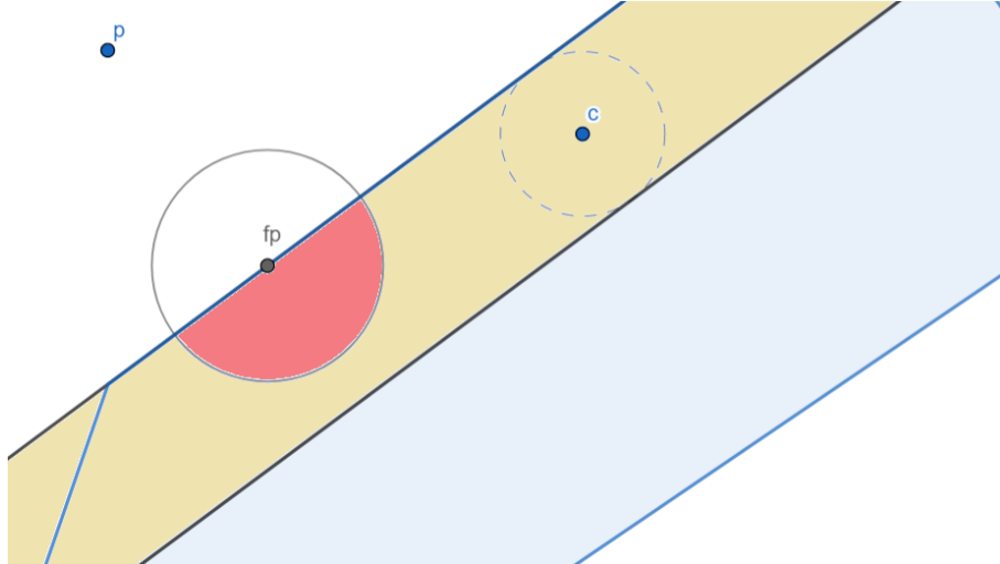
2.24. ábra. A gömbbel metszett henger (piros) A késsel keretezett rész a közelített felület, a sárga a közelítő henger
