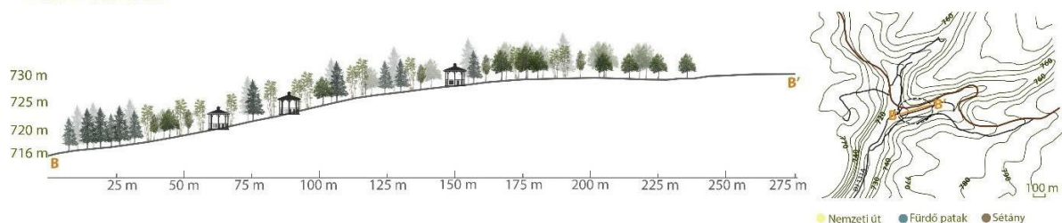
Hosszmetszet BB'
