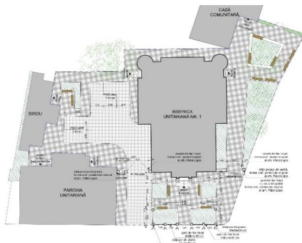
11 ábra- Javasolt helyszínrajz
