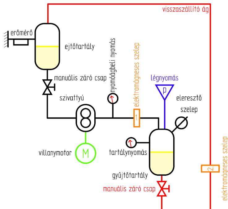
14. ábra A berendezés elvi vázlata
