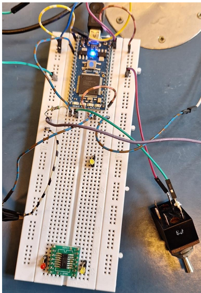
12. ábra A mikrokontroller tényleges kapcsolása. Középen az mbed LPC1768 kontrolller, felül a soros kommunikációt megvalósító számítógépes kapcsolathoz használt mini-USB kábel, jobb alul pedig a kitöltési tényező növelő kapcsoló látható.
