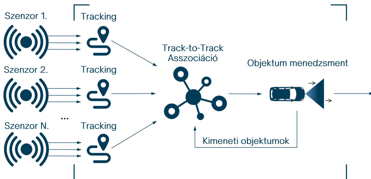
3.1. Ábra: Hibrid Track-to-Track architektúra visszacsatolással
