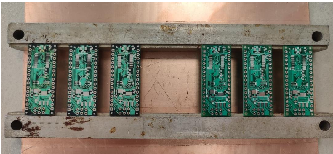
16.2.2. ábra: A HAST ciklus előtt (balra: lebomló; jobbra: FR4)
