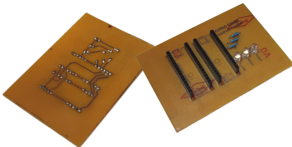
10.1.3. ábra: Az „otthoni módszerekkel” készített bootloader programozó áramkör.
