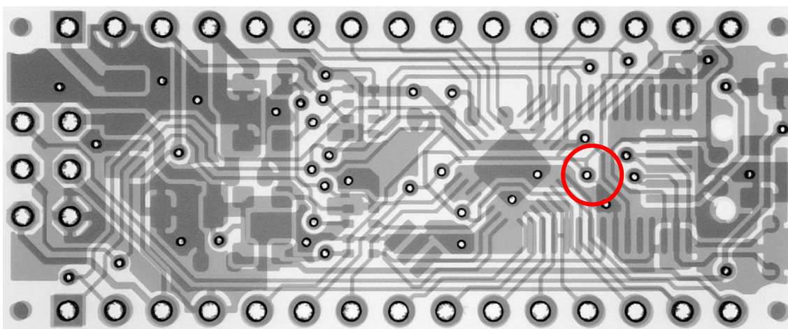
11.3.1. ábra: Röntgenkép egy rövidzárat tartalmazó áramkorról.
