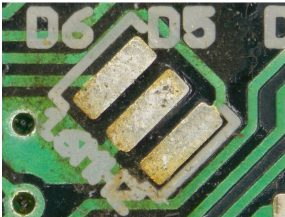
11.2.1. ábra: Lenolajjal erősen szennyezett forrasztási felület
