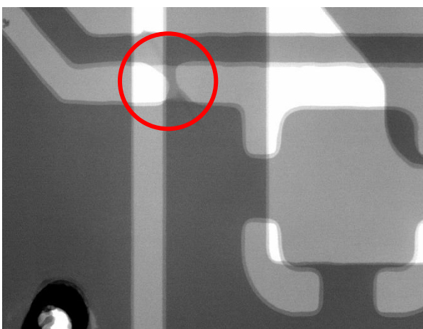
11.3.3. ábra: Rövidzár az RST és GND között
