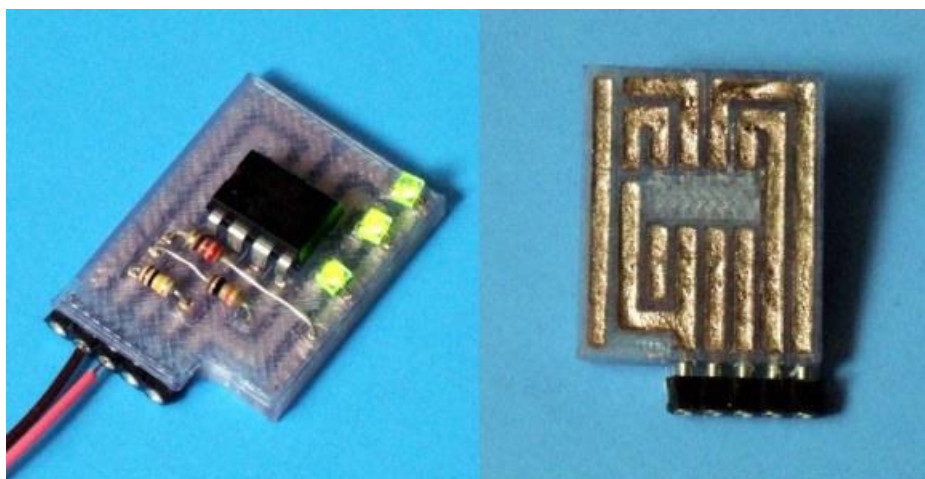
4.3.3. ábra: PLA alapú, forrasztásmentes, vezetékfestéssel bevont áramkör.[PIC_3]
