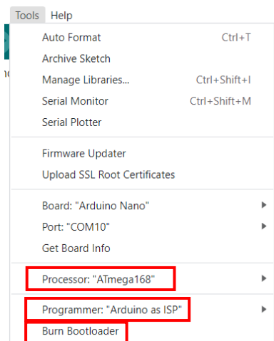
10.1.1. ábra: A bootloader égetéséhez szükséges menüpontok.
