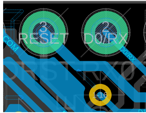
8.6. ábra: Korrigált furat-vezeték csatlakozás
