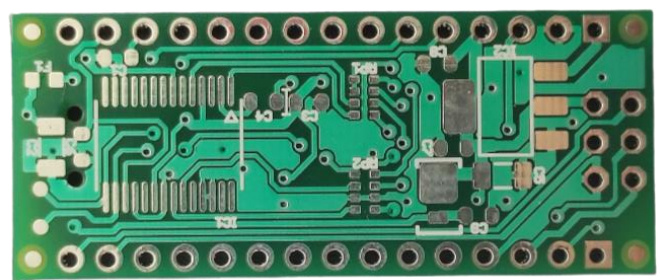
9.2. ábra: FR4-en létrehozott áramkör BOTTOM oldala
