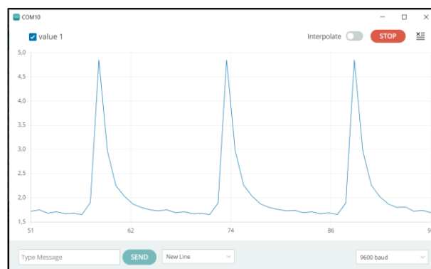
14.1.4. ábra: Soros porton kapott eredmény; tengelyek értékei: X: idő [s], Y feszültség [V]
