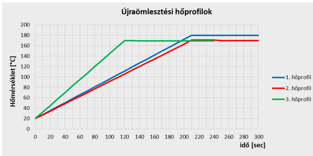
11.5.1. ábra: Tesztelt hőprofilok
