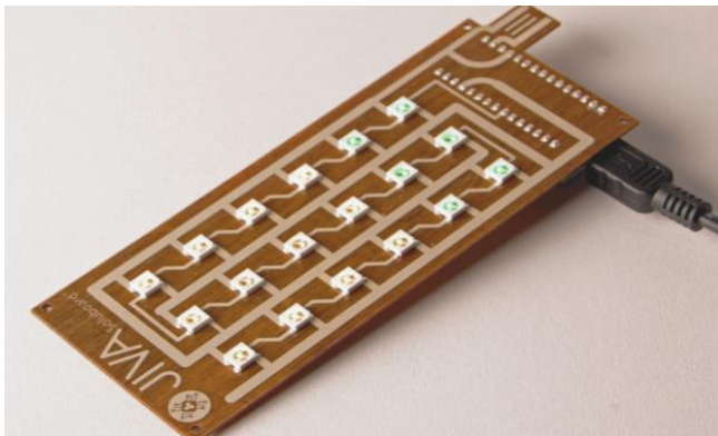
4.3.1. – 4.3.2. ábra: JIVA Soluboard®, melyről vízbe helyezve könnyen leszedhetők az alkatrészek, valamint megindul a rostokból készült hordozó delaminációja. [PIC_1][PIC_2]
