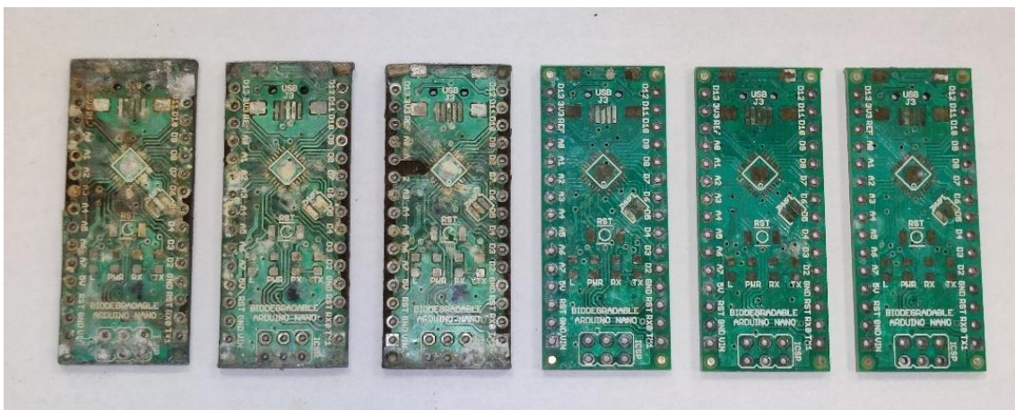
16.2.3. ábra: A HAST 6. ciklusa után (balra: lebomló; jobbra: FR4)
