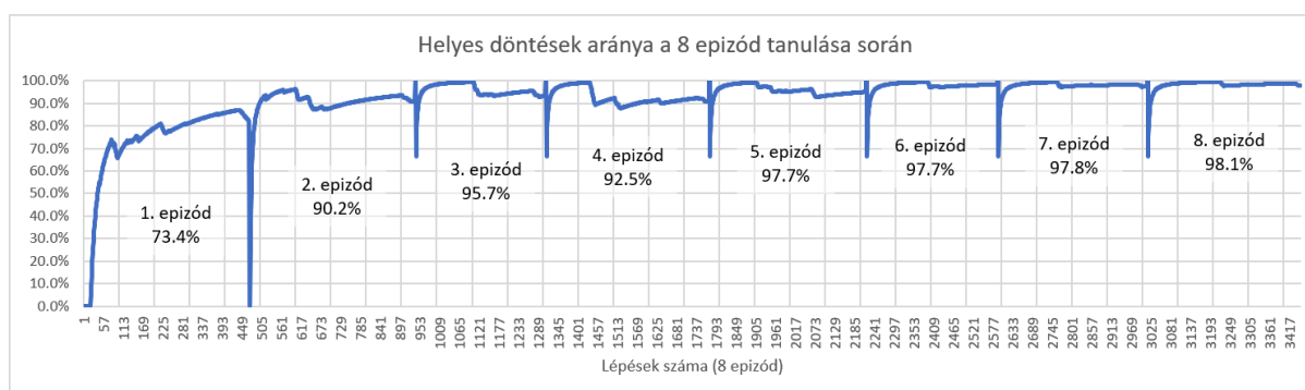
4.5-2. ábra: Az önvezető modul helyes döntéseinek aránya 8 epizódon keresztül
