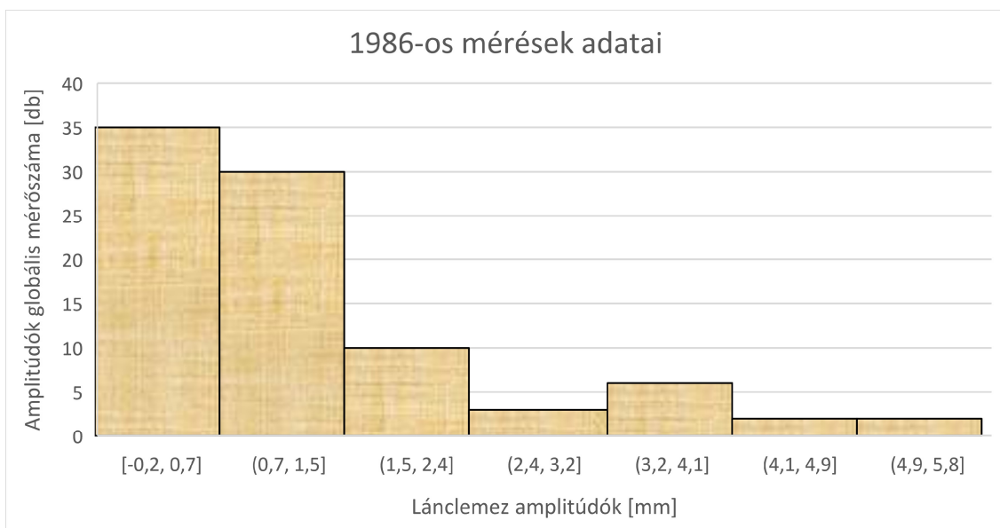
20. ábra: 1986-ban mért lánclemezvastagságok korróziós krátermélységei
