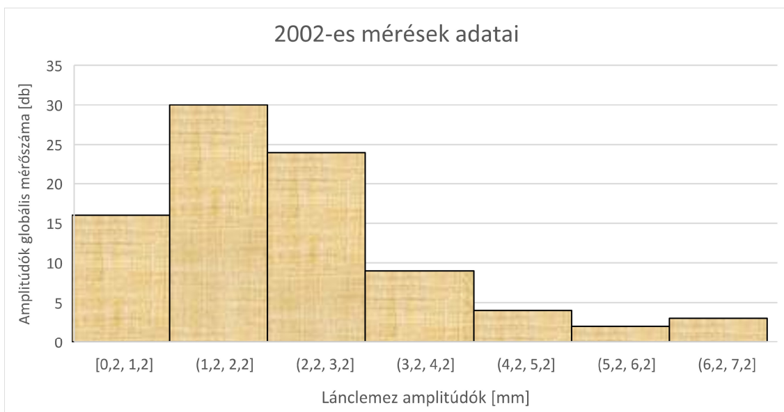
21. ábra: 2002-ben mért lánclemezvastagságok korróziós krátermélységei
