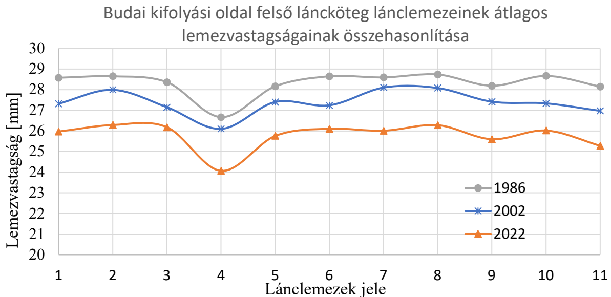
11. ábra: Budai kifolyási oldal felső láncköteg lánckötegeinek átlagos lemeztavastagságai
