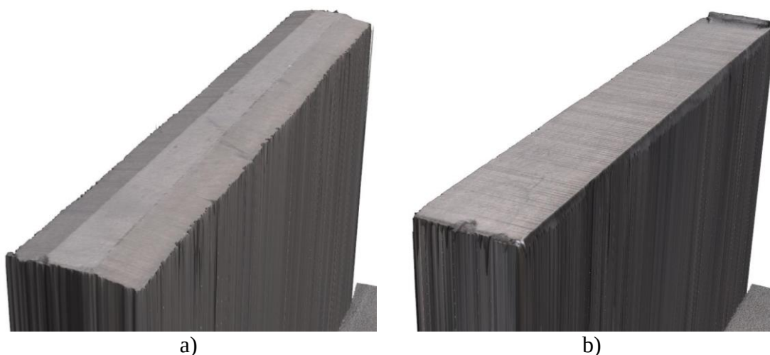
5.8. ábra A topográf-felület vizsgálatot meghatározott felületek ábrája, a) a legjobb felületi minőség, b) a legrosszabb felületi minőség
