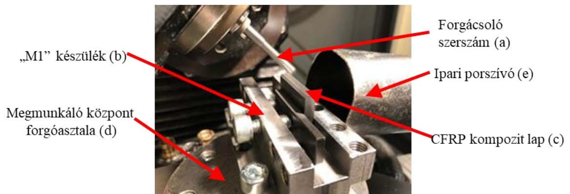
3.5. ábra Kísérleti környezet: (a) Forgácsoló szerszám, (b) „M1” munkadarab befogó készülék, (c) CFRP kompozit munkadarab, (d) Megmunkáló központ forgóasztala, (e) Ipari porszívó
