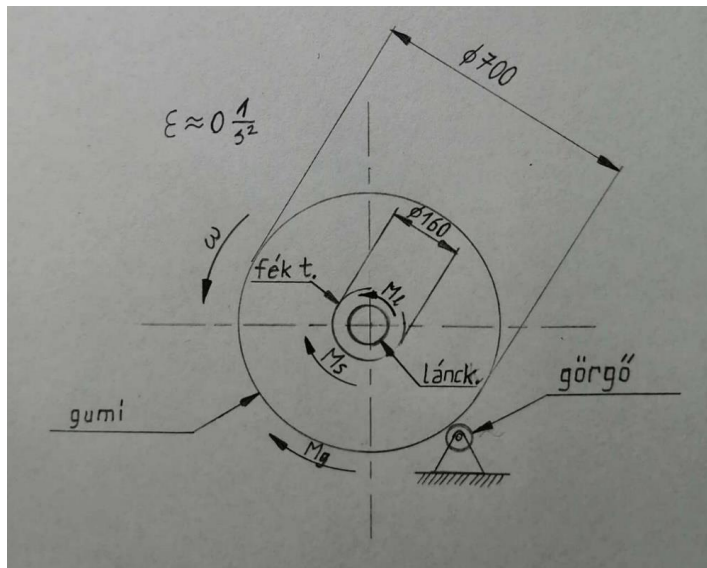
13. Ábra: A hátsó kerék egyszerűsített modellje
