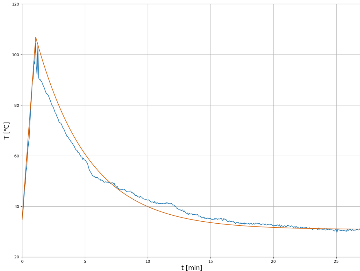
7. Diagram: Féktárcsa melegedése és hűlése Első mérés második fékezés Késsel: mérés Sárgával: szimuláció
