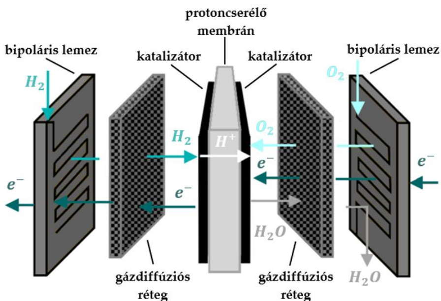
1. ábra A hidrogéncella felépítése [12] alapján
