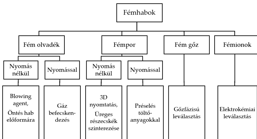
5. ábra Fémhab gyártási technológiák csoportosítása [36] alapján
