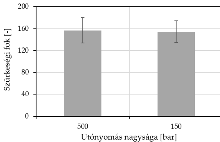
22. ábra Az utónyomás hatása a minták szürkeségi fokára
