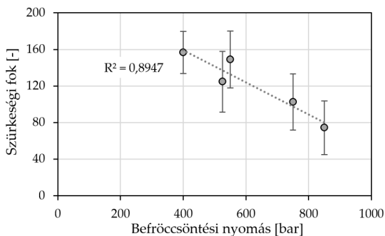
21. ábra A minták szűrkeségi foka a befroccsöntési nyomás függvényében
