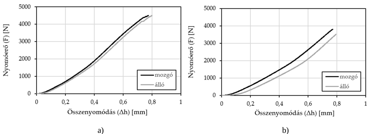
28. ábra A 4. (a) és a 8. (b) hab nélküli minta benyomódása
