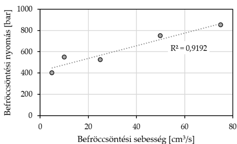
19. ábra Az alkalmazott befroccsöntési sebesség és befroccsöntési nyomás kapcsolata
