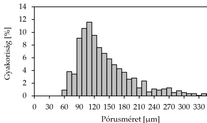
15. ábra Az automatikus mérés pórusméreteloszlása (nagyítás 40×)
