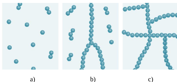
6. ábra Termikus perkoláció mechanizmusa a töltőanyag növelésével [51]
