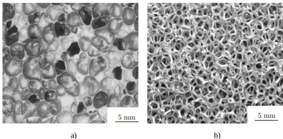
4. ábra Zárt (a) és nyílt (b) cellás alumínium hab szerkezete [38]
