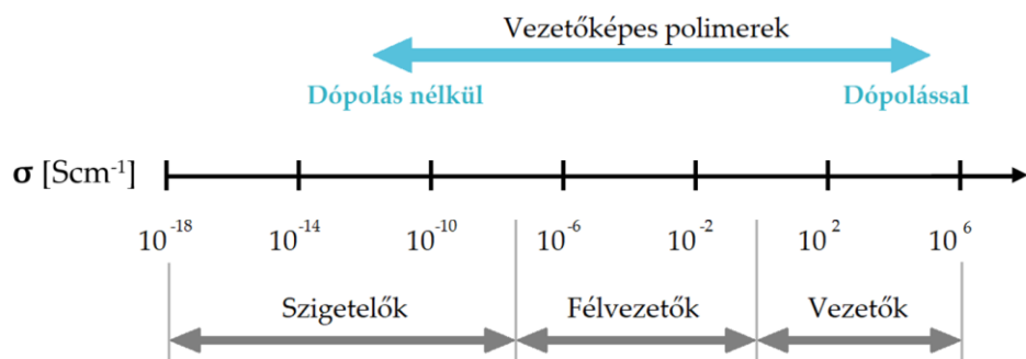
7. ábra Anyagsaládok csoportosítása az elektromos vezetőképesség szerint [56] alapján
