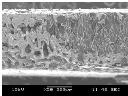
35. ábra Az ömledékfront és az áramlás irányában elhelyezett fémhab találkozása
