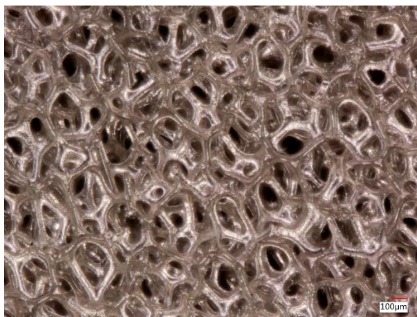
13. ábra A nyílt cellás nikkelfab szerkezete (nagyítás 100×)
