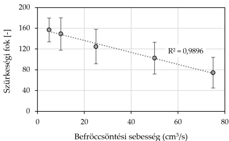
20. ábra A minták szűrkeségi foka a befroccsöntési sebesség függvényében
