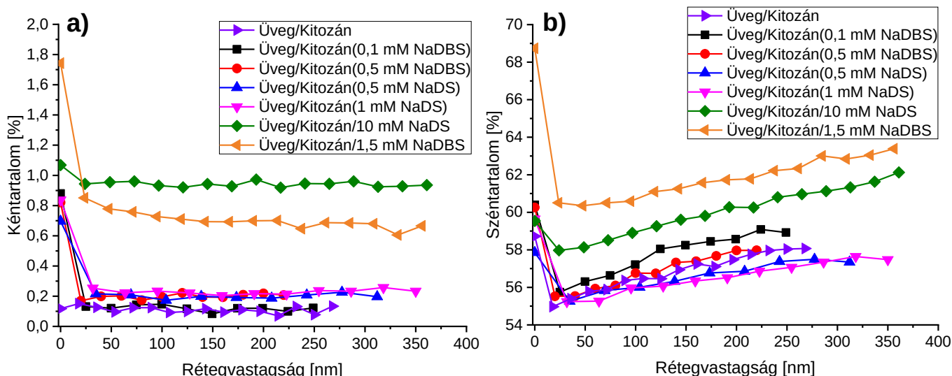
22. ábra: A tenzidtartalmú bevonatok a) kén- és b) széntartalma a rétegvastagság függvényében
