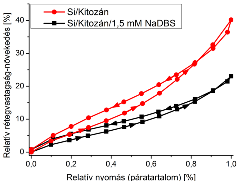
25. ábra: A natív (kémiailag nem módosított) és 1,5 mM NaDBS-el impregnált bevonatok vízgőzfelvételének változása a relatív páratartalom függvényében (a görbéken látható nyilak mutatják, hogy az adott pontok a duzzadás, azaz a pártartalom növelésének szakaszában, vagy a száradás szakaszában lettek felvéve).
