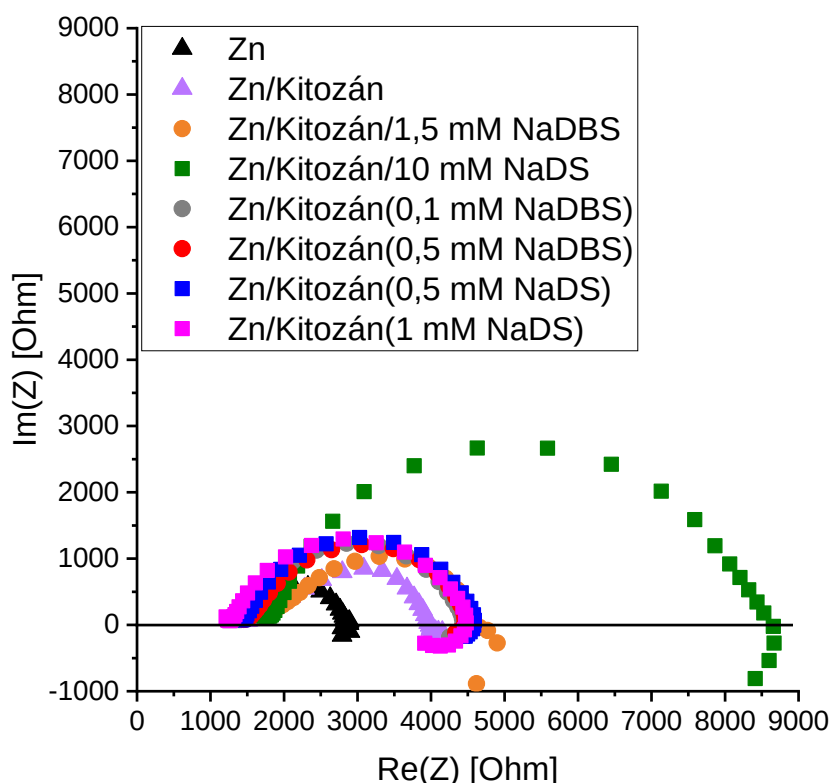
24. ábra: Az összes vizsgált minta impedanciaspektruma 0,2 g/l-es \text{Na}_2\text{SO}_4 elektrolitban vizsgálva. A spektrumon megjelenő félkör átmérője arányos a vizsgált rendszer polarizációval szembeni ellenállásával.
