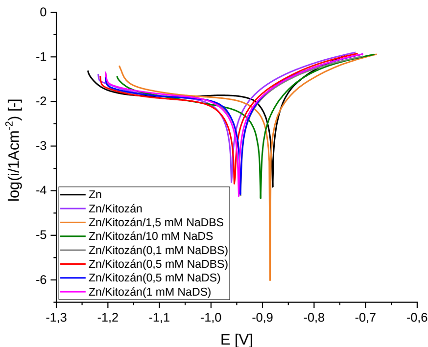
23. ábra: Az elektrokémiai polarizációs tesztek eredménye képpen kapott Tafel-görbék az összes vizsgált rendszer esetén 0,2 g/l-es Na_2SO_4 elektrolitban vizsgálva
