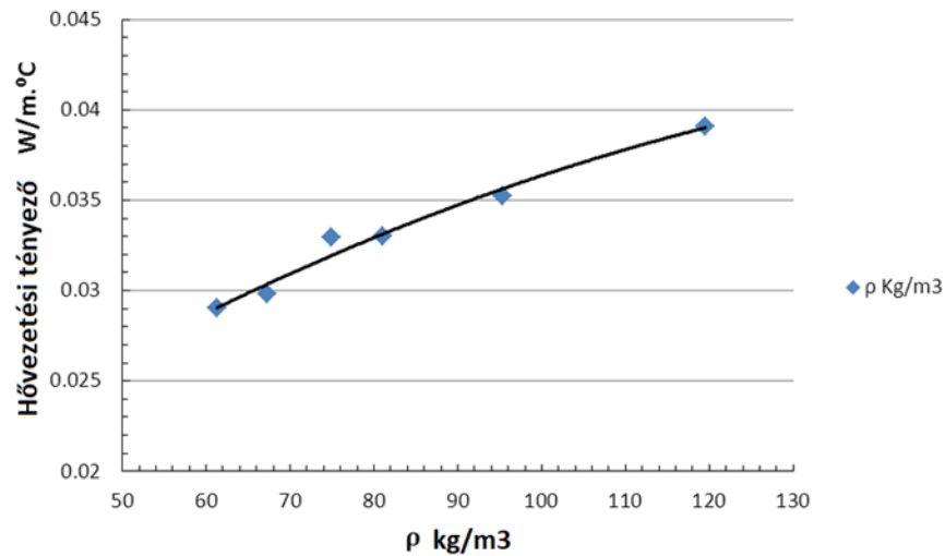
1.ábra: Üveggyapot hővezetési tényezőjének változása a sűrűség függvényében [2]
