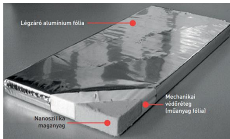
9.ábra: Vákuumpanel felépítése [14]
