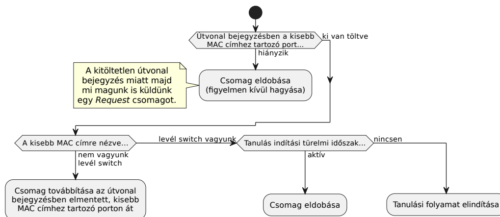
3.14. ábra. Request csomagok feldolgozásának algoritmususa
