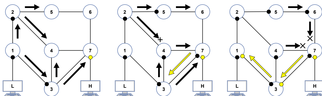
3.9. ábra. Tanulási algoritmus működése köröket tartalmazó hálózatban. Az útvonal az L és a H hosztokhoz tartozó levél switchek között kerül kiépítésre, ahol L a kisebb MAC címmel rendelkező hoszt. A fekete nyilak Learn , a sárga nyilak pedig Confirmation csomagokat jelölnek. A keresztkben végződő nyilak a csomagok eldobását jelzik. A portokhoz tartozó pöttyök pedig a megtanult portokat szimbolizálják.
