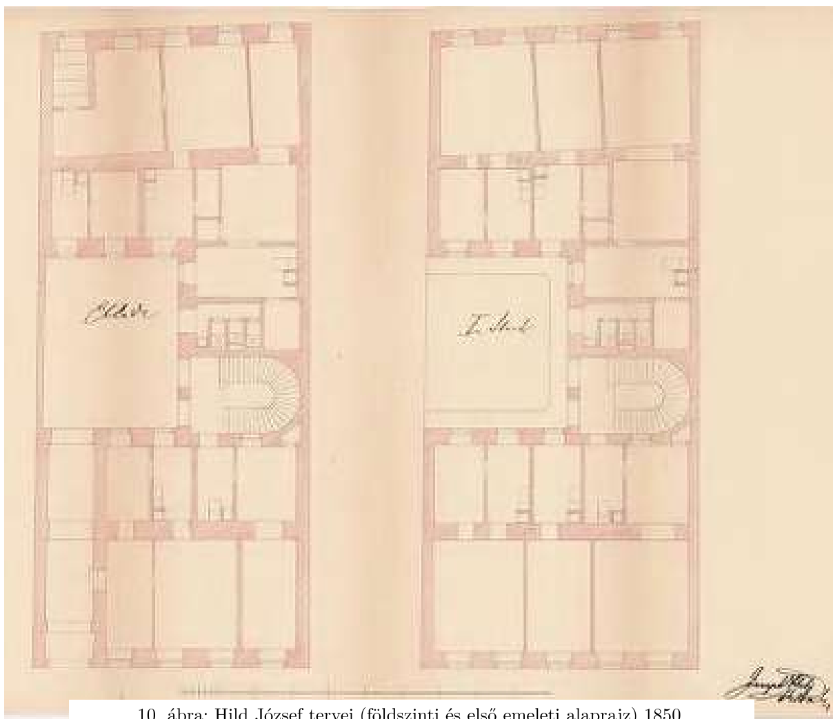
10. ábra: Hild József tervei (földszinti és első emeleti alaprajz) 1850.
