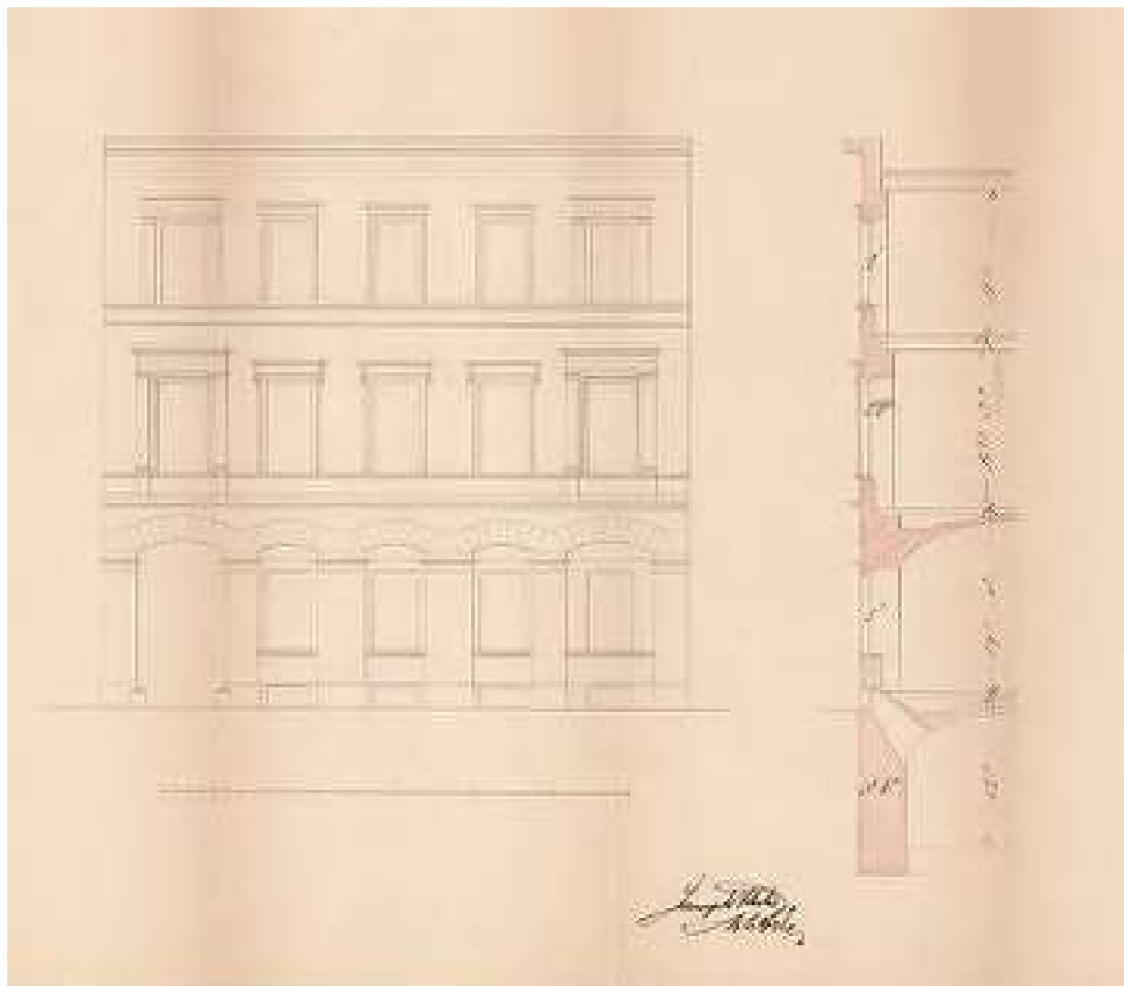
11. ábra: Hild József tervei (homlokzat, metszet) 1850
