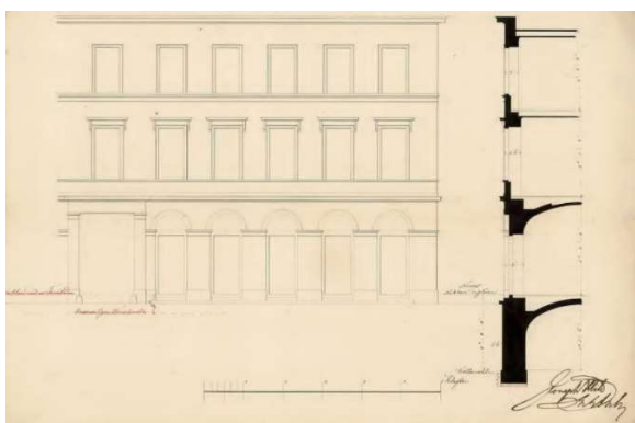
16. ábra: Andrássy út 9. sz. ház homlokzatterve, Hild József, 1840 (Építtető: Michl János).
