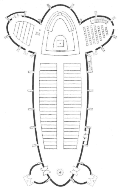
a frankfurti St. Michael eredeti metszete, alaprajza
