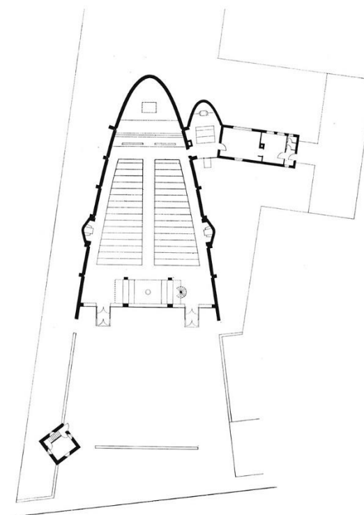
a bottropi Heilig Kreuz templom alaprajza
