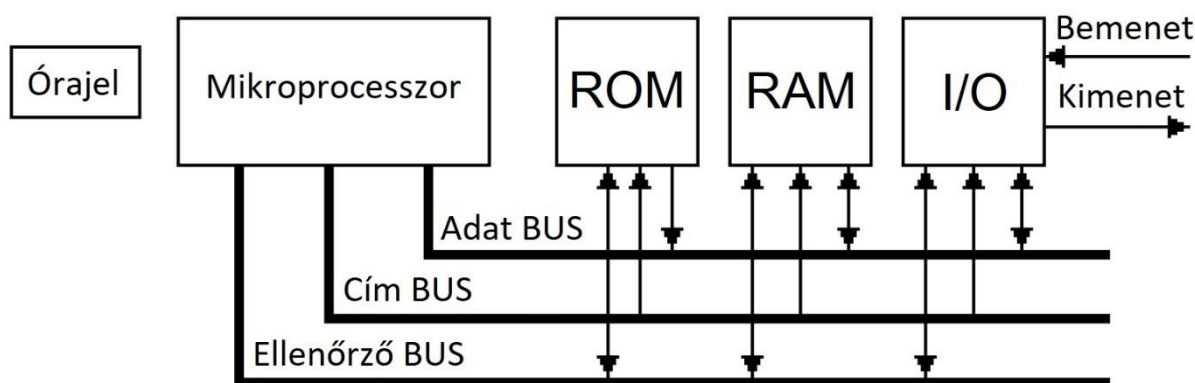
29. ábra: Mikroszámítógép felépítése
