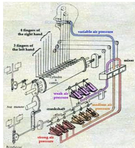
1. ábra: Fuvolajátékos mechanikája
