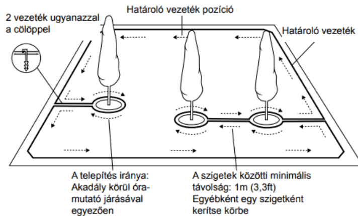
16. ábra: A robotfűnyíró területének behatárolása
