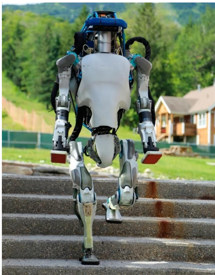
26. ábra: Lépcsőn lesétáló Boston Dynamics (forrás: https://robotsguide.com/robots/atlas2016 )
