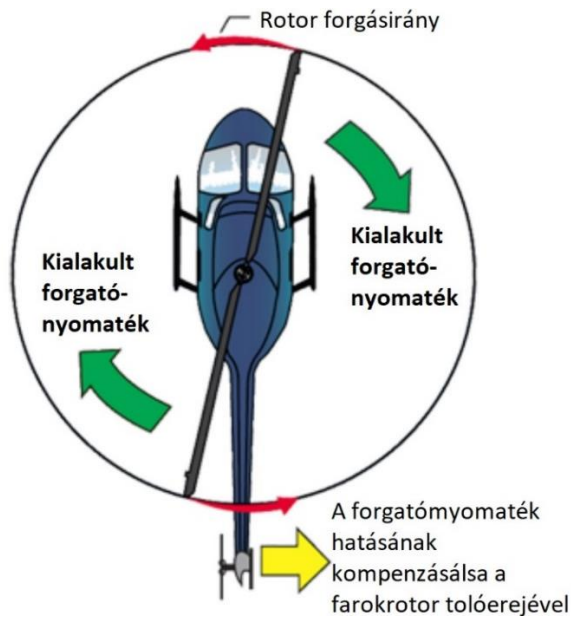
24. ábra: Helikopter farokrotorjának kiegyenlítő hatása
