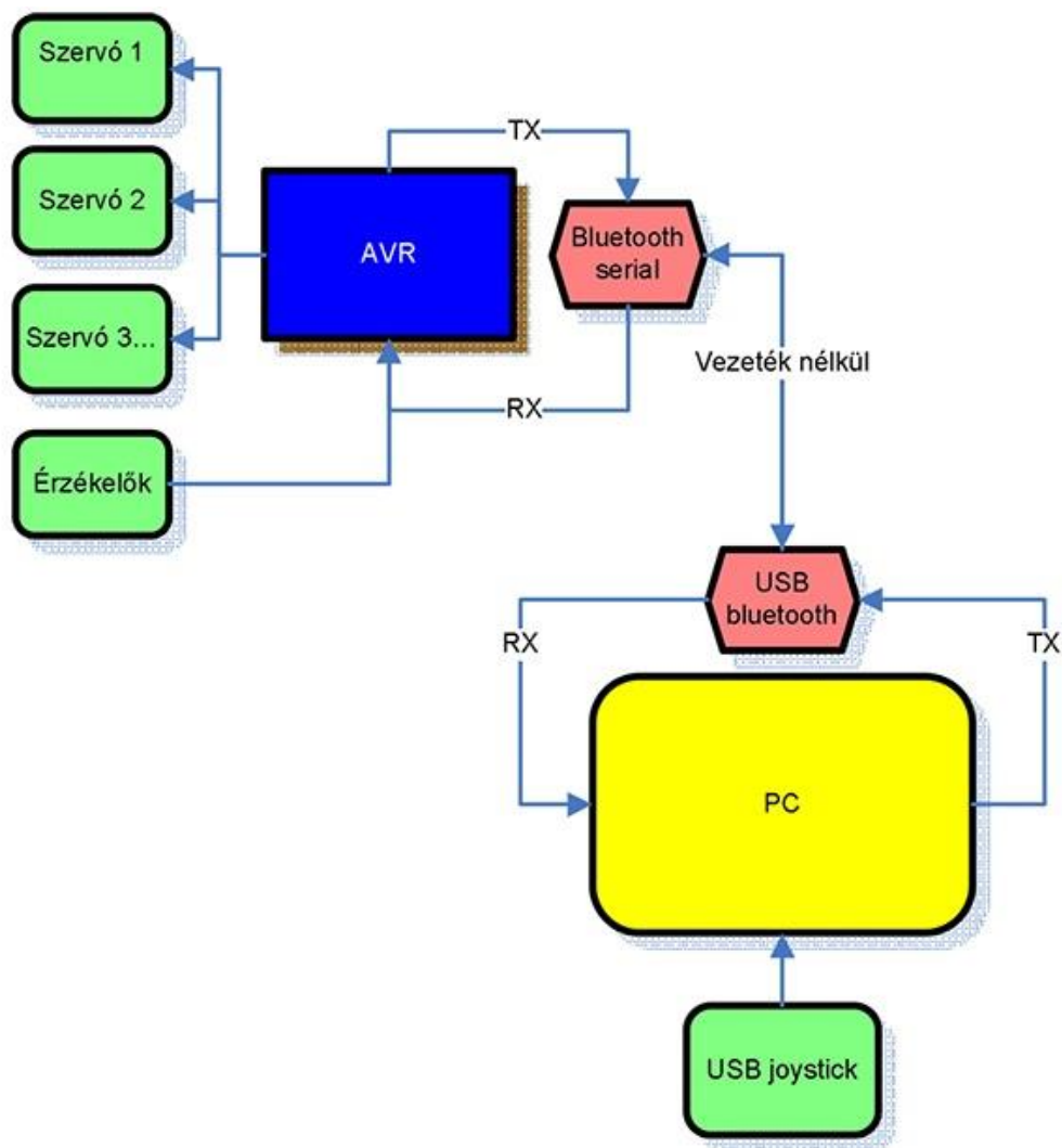
23. ábra: Hatlábú robot folyamatabrája
