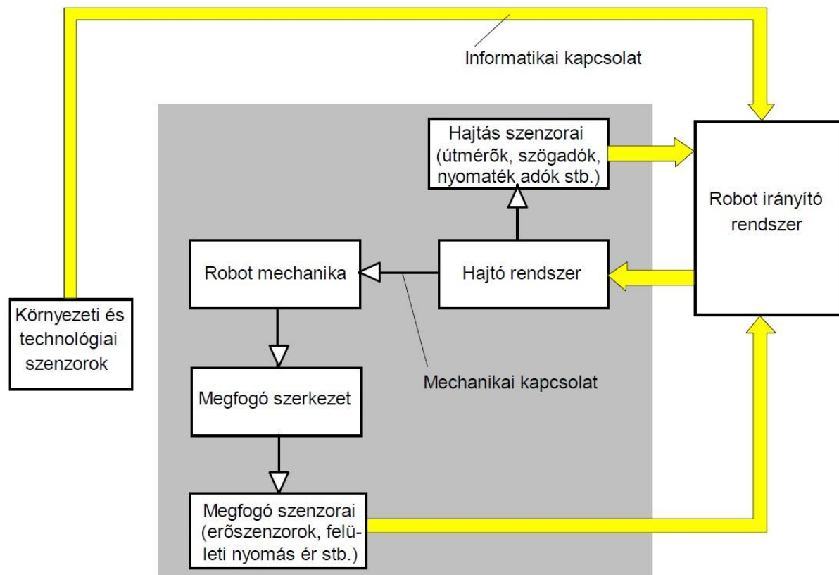
13. ábra: A robot funkcionális egységei
