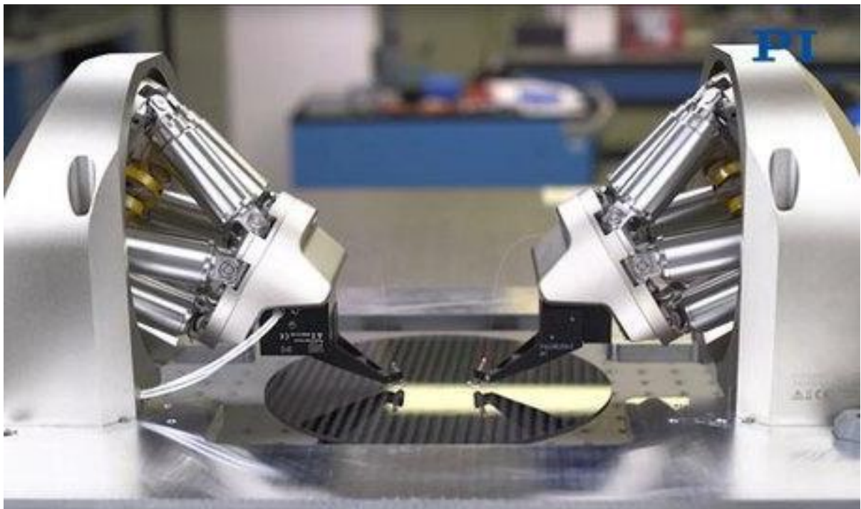
19. ábra: Félvezető gyártó hexapod
