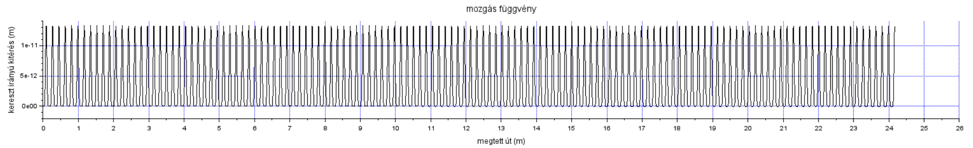
2-es melléklet 3. ábra: A golyó mozgása szűkített tartományban, \omega_\psi = 84,5 \frac{1}{s} ; \omega_\theta = 1 ; \omega_\phi = 0
