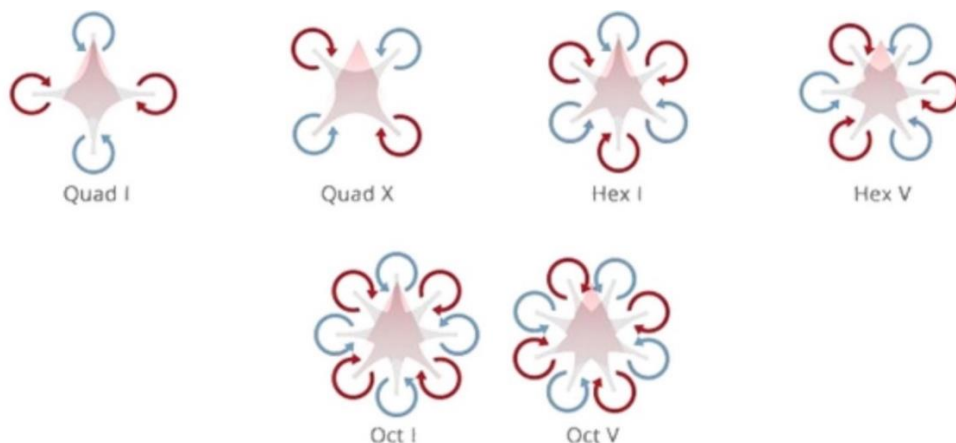
25. ábra: Multikopterek rotorszám alapján
