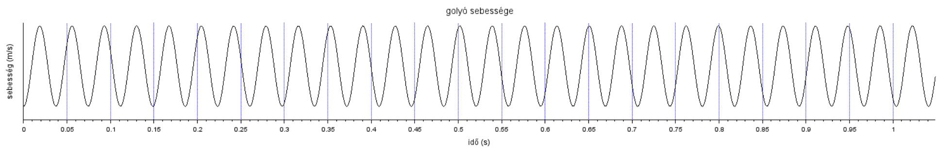
5. számú melléklet 3. ábra: A golyó mozgása szűkített tartományban, \omega_\psi = 84,5\frac{1}{s} ; \omega_\theta = 1 ; \omega_\phi = 0
