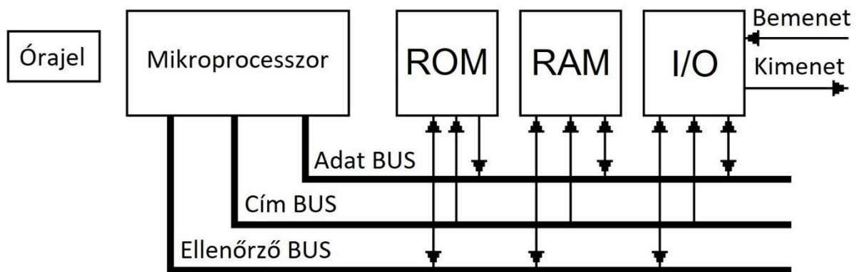
3. számú melléklet 1. ábra: Mikroszámítógép felépítése
