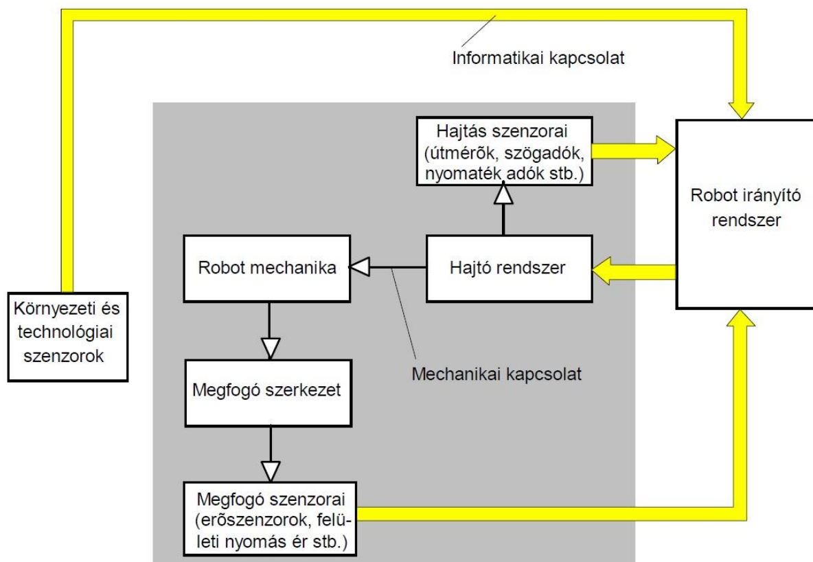
1. melléklet 13. ábra: A robot funkcionális egységei
