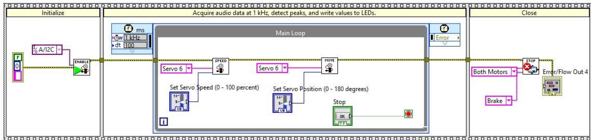
6. számú melléklet 4. ábra: Behatárolt forgású szervomotor vezérlése
