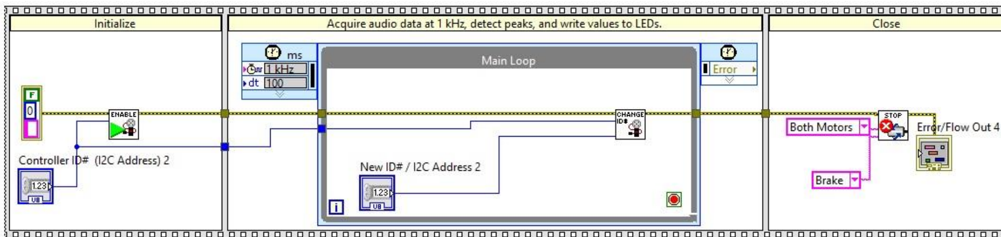
6. számú melléklet 2. ábra: A szervomotorok azonosítása
