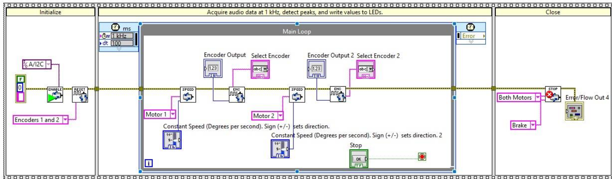
6. számú melléklet 3. ábra: A DC motorok vezérlése
