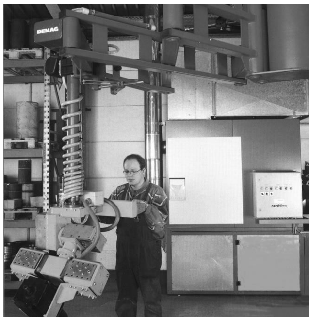
1. melléklet 11. ábra: Nagyteherbírású manipulátor programozása (forrás: Kulcsár Béla, Robottechnika [2012])
