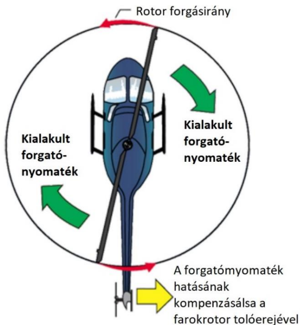
2. melléklet 11. ábra: Helikopter farokrotorjának kiegyenlítő hatása
