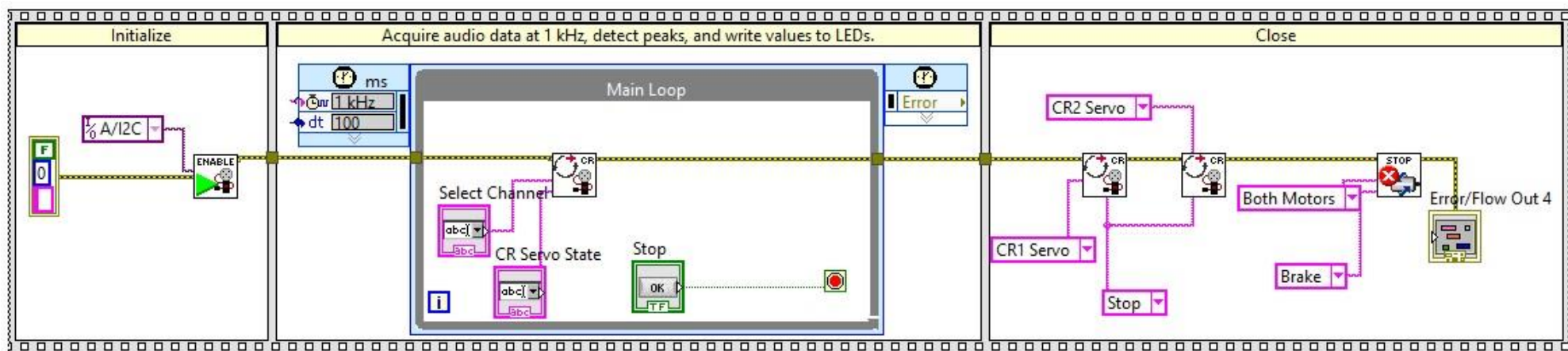
6. számú melléklet 5. ábra: Folyamatos körbefordulású szervomotor vezérlése
