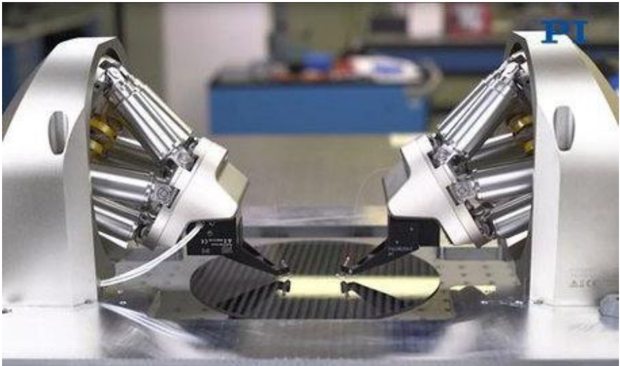
2. melléklet 6. ábra: Félvezető gyártó hexapod
