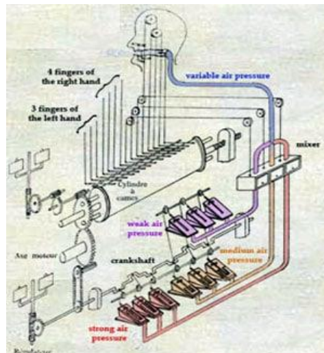
1. melléklet 1. ábra: Fuvolajátékos mechanikája
