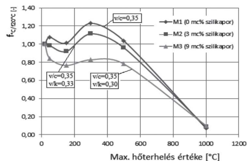
7. ábra Azonos v/c tényezőjű keverékek maradó relatív nyomószilárdság átlagértékei Fig. 7. Relative residual compressive strength with constant v/c ratio
