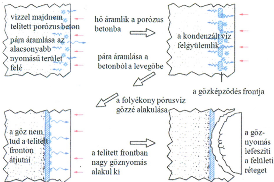
3. ábra: A beton felület leválásának mechanizmusa [11]
