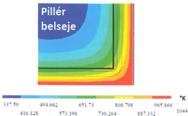
5. ábra: Ansys modell 120 perces hőterhelés hatására kialakuló betonhőmérséklet eloszlásáról egy vasbeton pillér élénél
