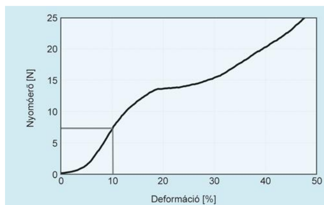
4. ábra. A nyomóerő változása a deformáció függvényében
